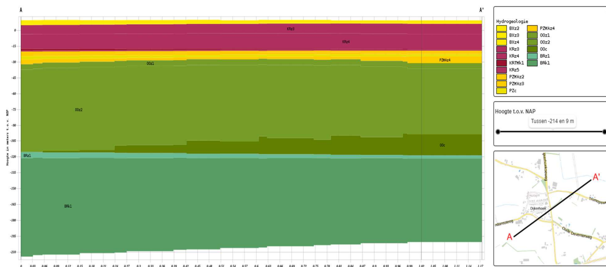
figuur 3: de geohydrologische opbouw
