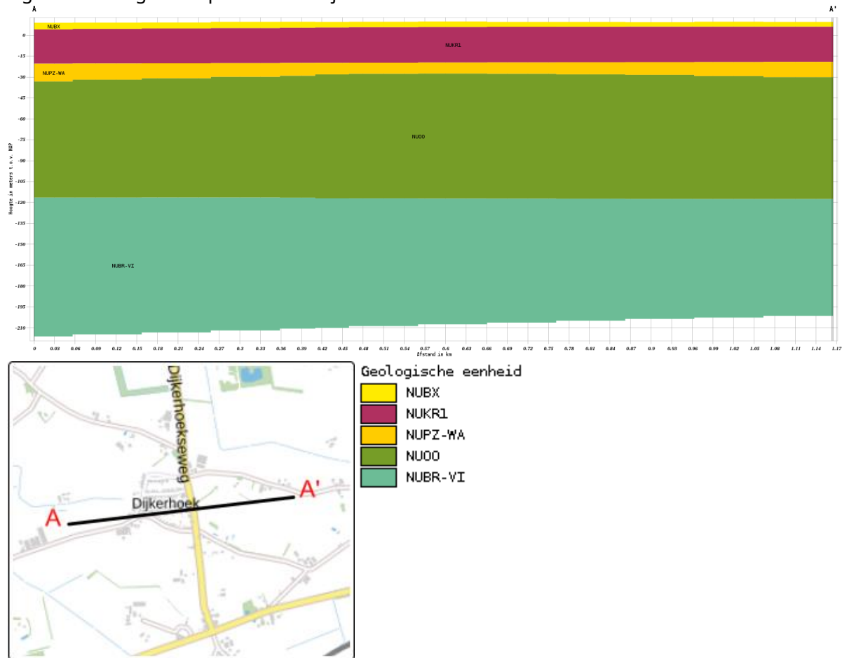
Figuur 1 Geologische opbouw landelijk model DGM v2.2
