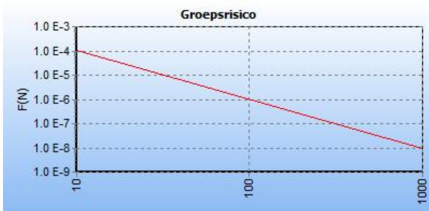
5.8 Figuur 5.8 FN curve voor A-806 van N.V. Nederlandse Gasunie voor de kilometer tussen stationing 16140.00 en stationing 17140.00
