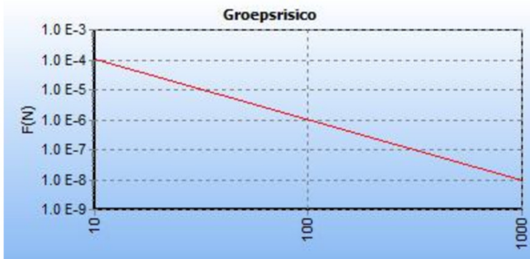
5.7 Figuur 5.7 FN curve voor A-662 van N.V. Nederlandse Gasunie voor de kilometer tussen stationing 12150.00 en stationing 13150.00
