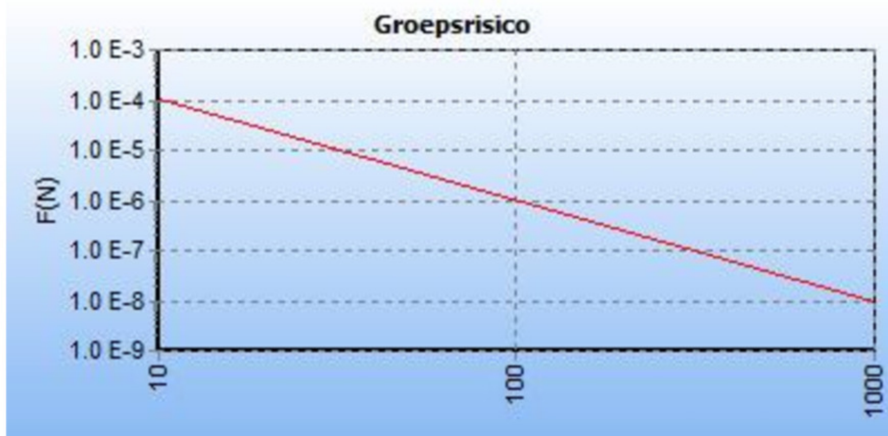
5.4 Figuur 5.4 FN curve voor A-529 van N.V. Nederlandse Gasunie voor de kilometer tussen stationing 23900.00 en stationing 24900.00
