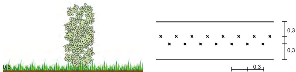
Afbbeelding 46. Dwarsprofiel en beplantingsschema strakke haag (maten in meters)
