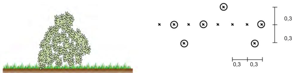
Afbbeelding 45. Dwarsprofiel en beplantingsschema losse haag (maten in meters)
