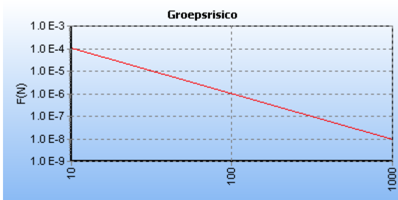
5.2 Figuur 5. 2 FN curve voor N-557-52 van N.V. Nederlandse Gasunie voor de kilometer tussen stationing 0.00 en stationing 1000.00
