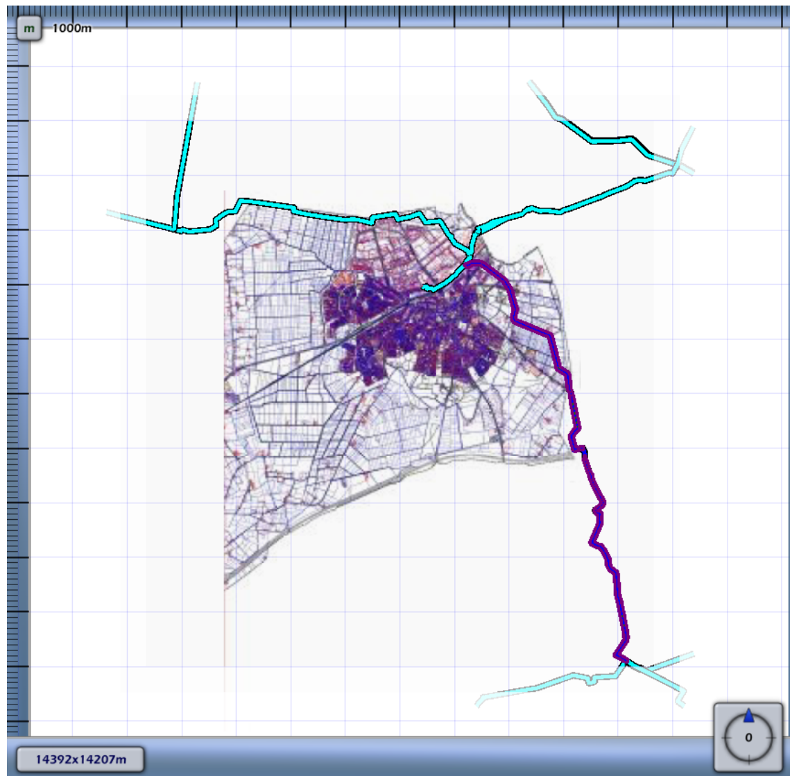
3.2 Figuur 3. 2 Plaatsgebonden risico voor N-557-52 van N.V. Nederlandse Gasunie
