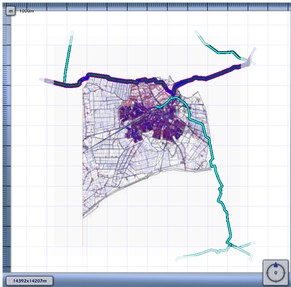
3.1 Figuur 3.1 Plaatsgebonden risico voor N-557-30 van N.V. Nederlandse Gasunie
