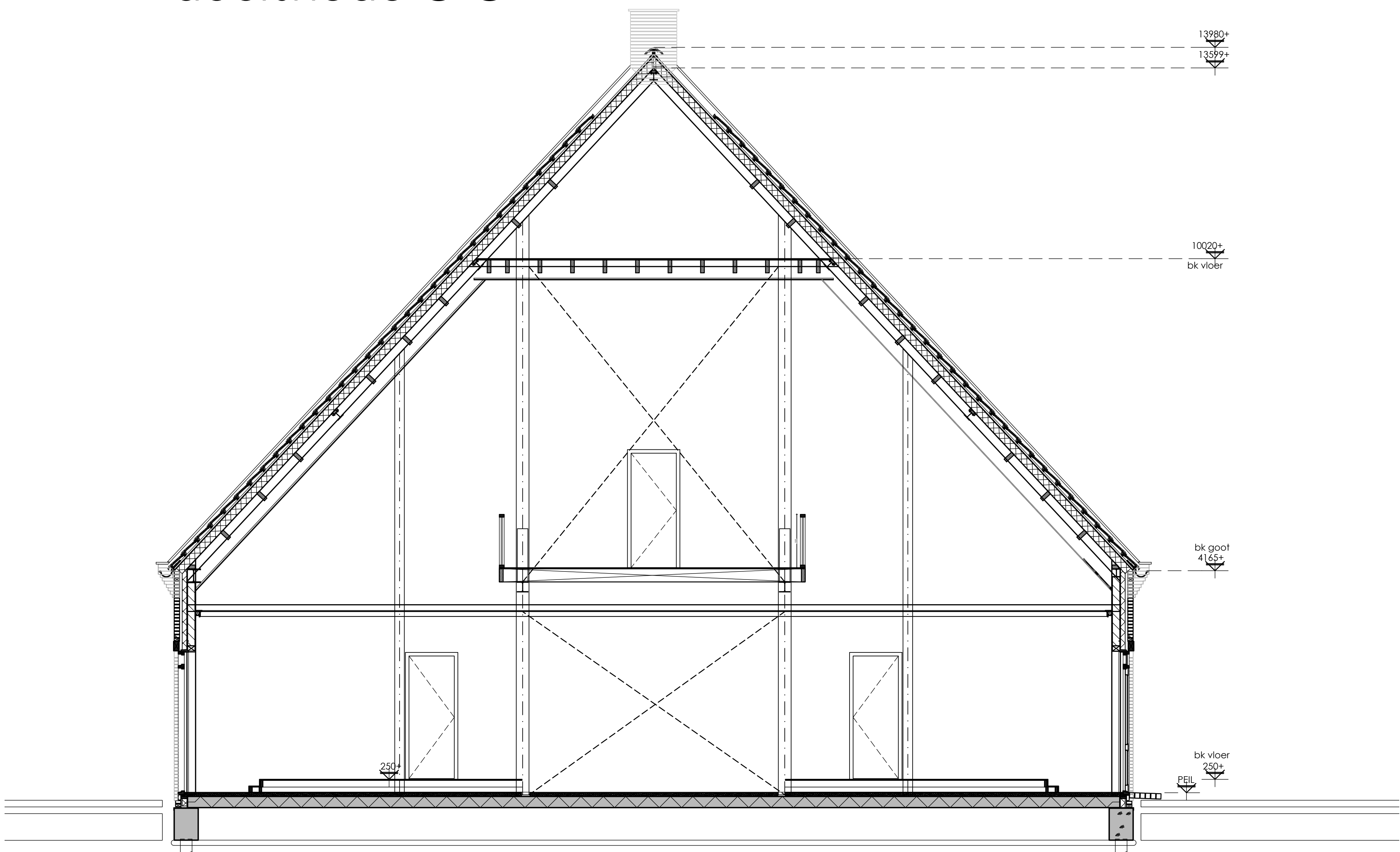
doorsnede C-C
