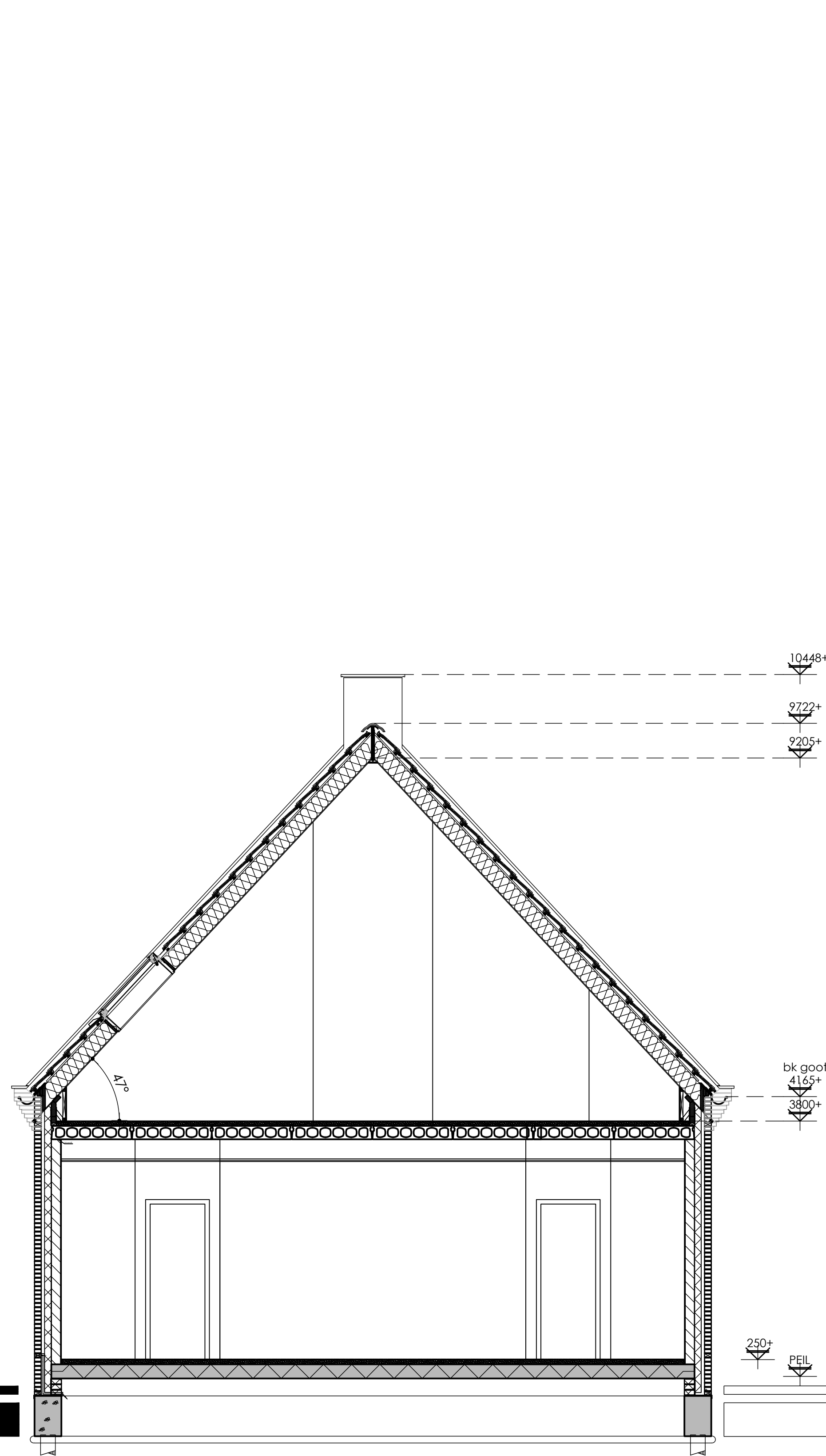
doorsnede B-B
