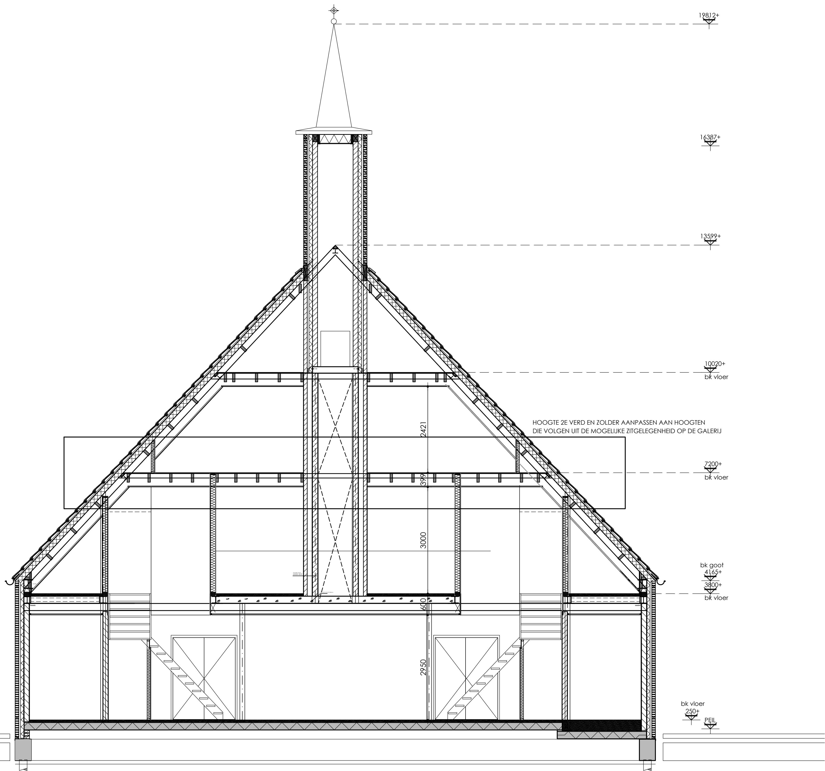
doorsnede C-C
