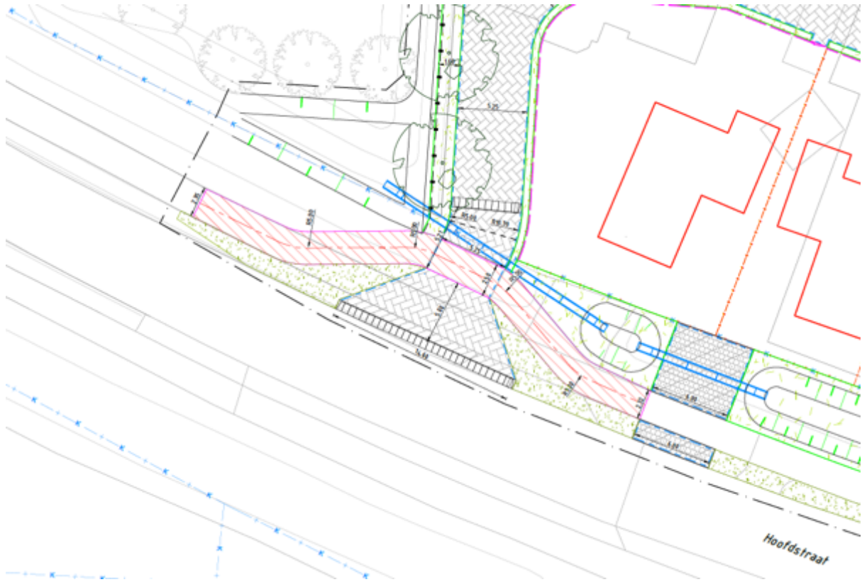
Afbeelding 4.1.: Inrichtingstekening met daarop de nieuwe inrit van het bouwplan op de Hoofdstraat.
