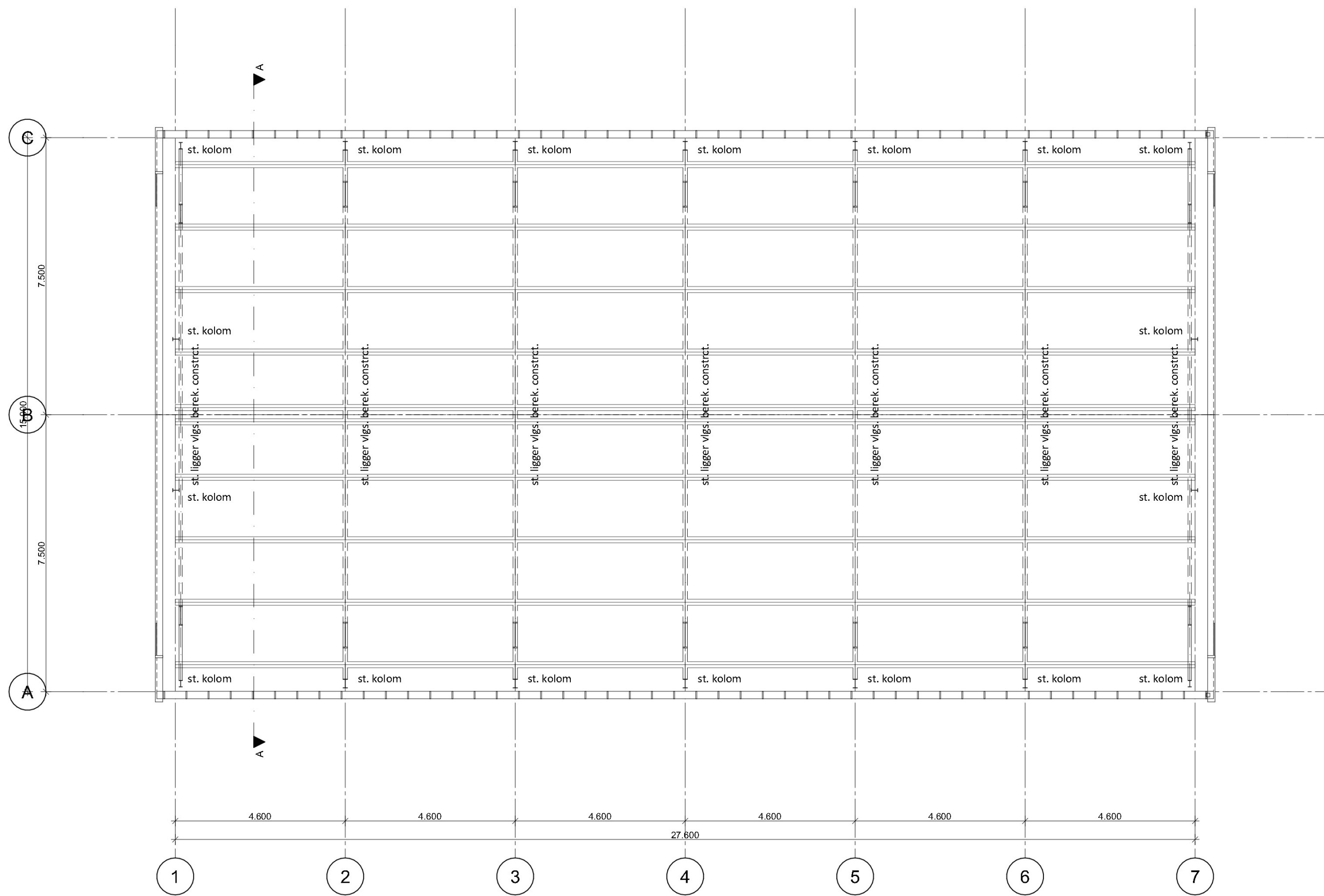
Kapplan
