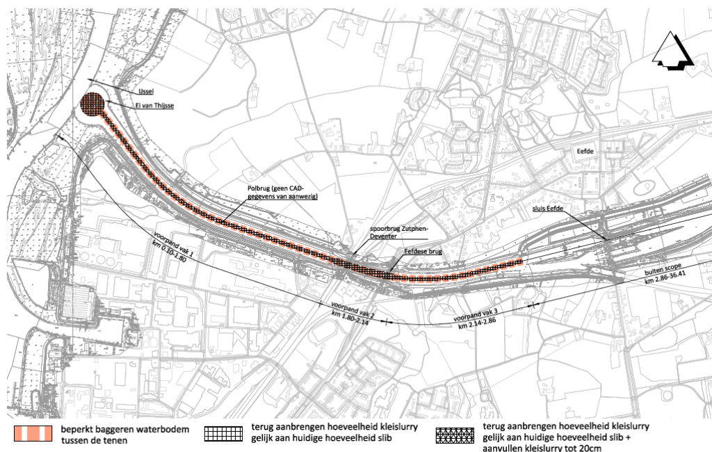
Figuur 2-2: Overzicht voorpand IJssel-Eefde
