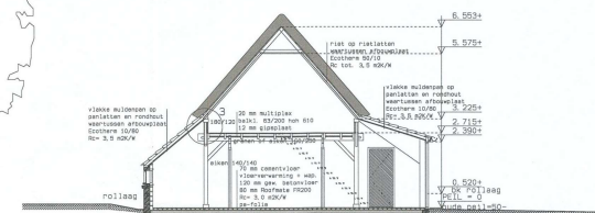
doorsnede C-D
