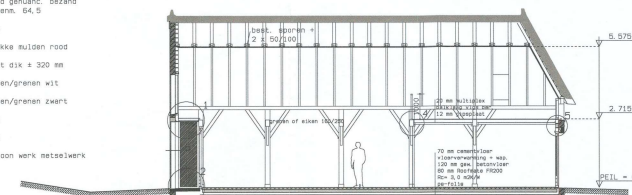
doorsnede E-F
