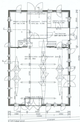
plattegrond
