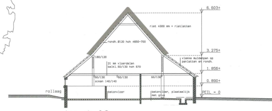
doorsnede C-D
