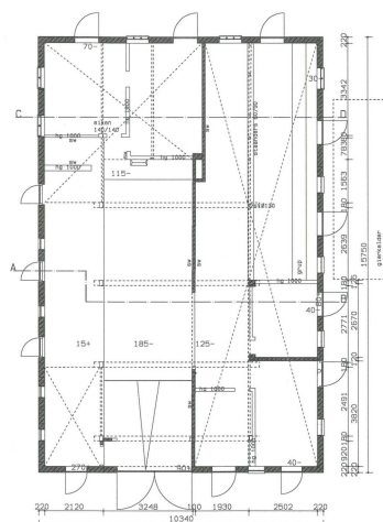
plattegrond
