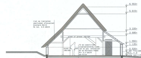
doorsnede A-B
