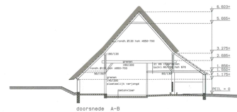
doorsnede A-B
