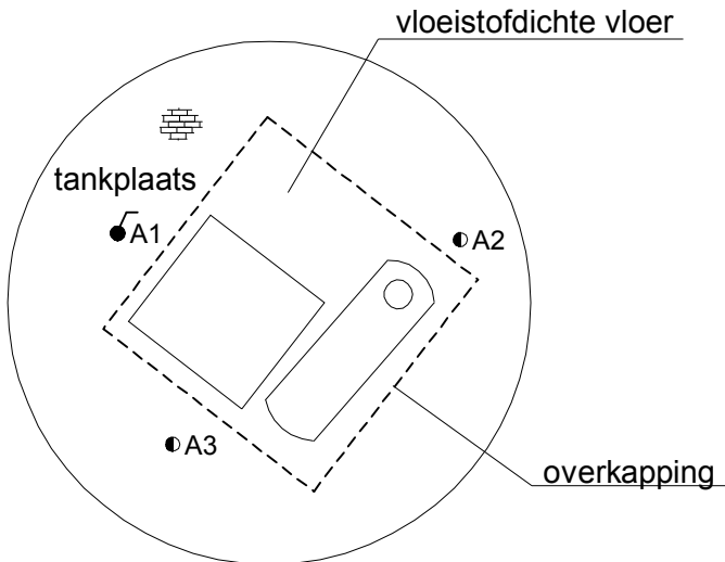
Detailtekening Deellocatie A Schaal 1 : 100
