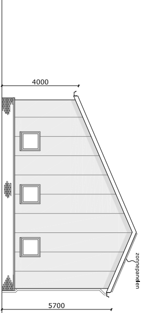
LINKER ZIJGEVEL (rechter zijgevel is spiegelbeeld)
