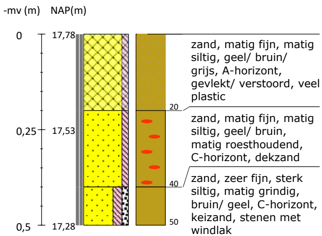
Boring 7 RD-coördinaten: 229856/475599
