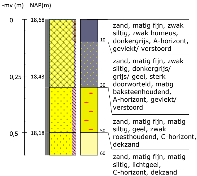
Boring 7 RD-coördinaten: 229856/475599
