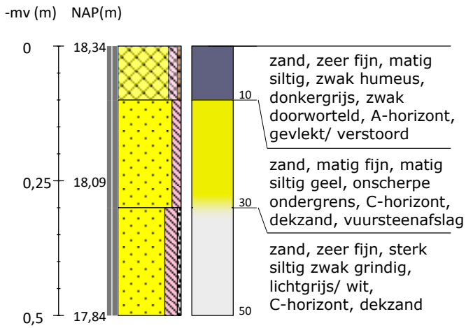
Boring 11 RD-coördinaten: 229918/475600
