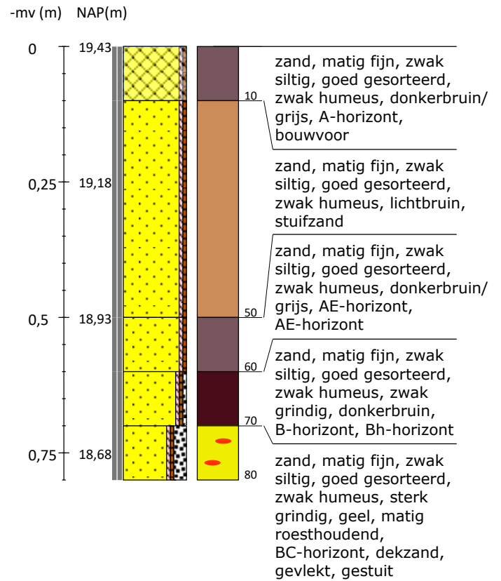
Boring 30 RD-coördinaten: 229941/475553
