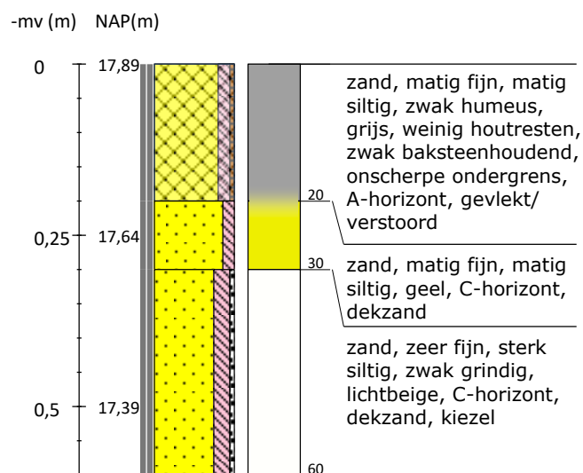
Boring 2 RD-coördinaten: 229868/475613
