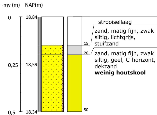
Boring 11 RD-coördinaten: 229918/475600
