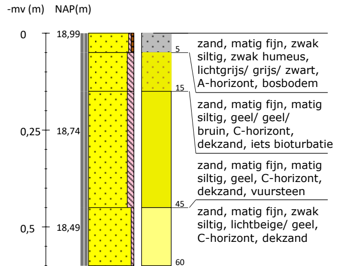
Boring 6 RD-coördinaten: 229922/475607
