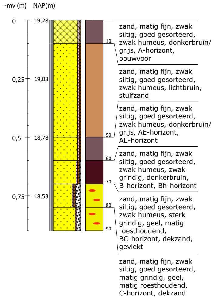
Boring 38 RD-coördinaten: 229961/475540
