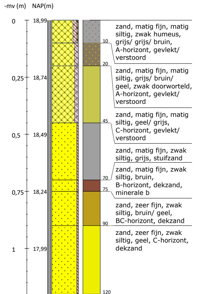
Boring 12 RD-coördinaten: 229930/475597
