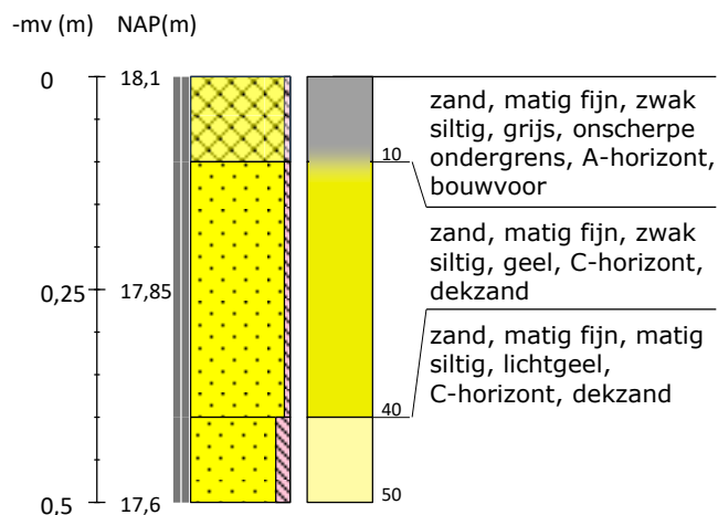
Boring 3 RD-coördinaten: 229879/475612
