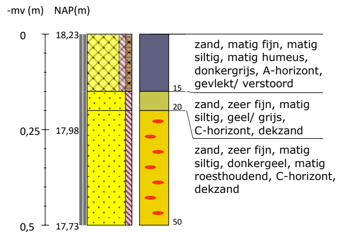
Boring 8 RD-coördinaten: 229871/475598
