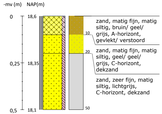
Boring 12 RD-coördinaten: 229930/475597
