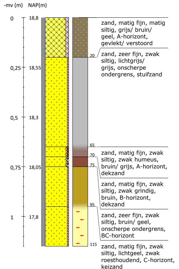
Boring 18 RD-coördinaten: 229943/475584
