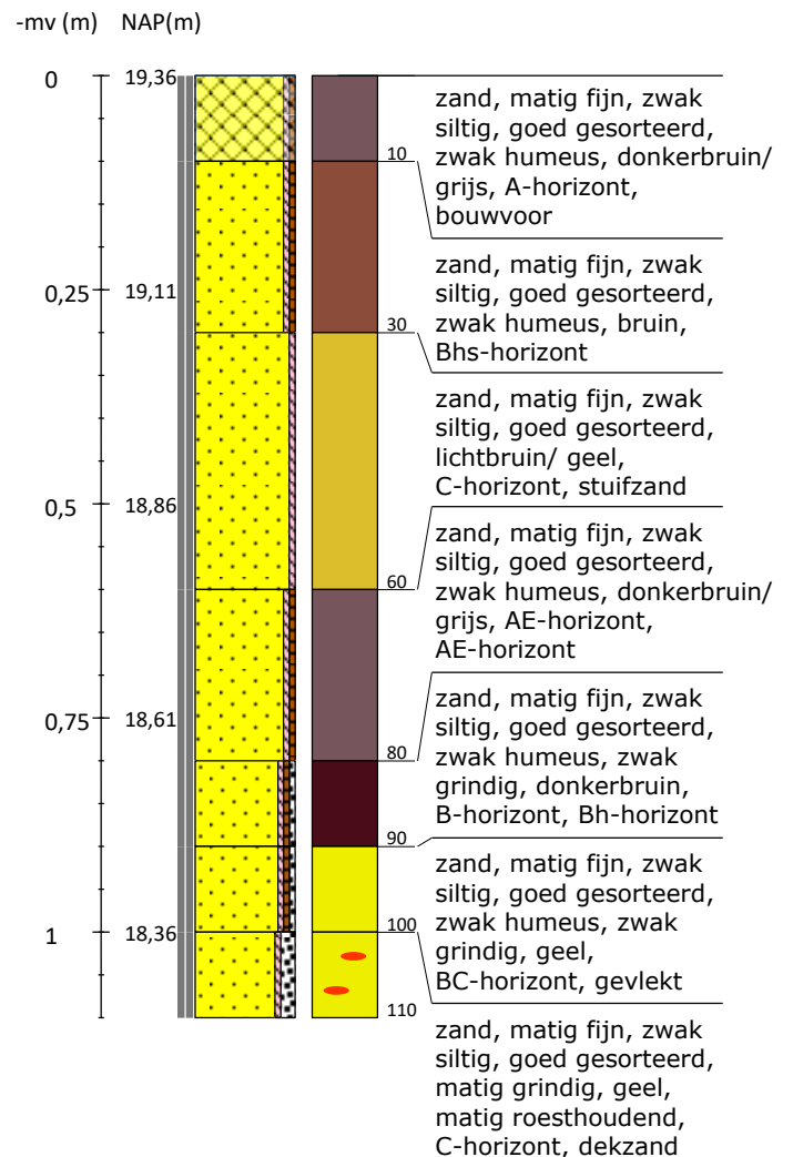
Boring 24 RD-coördinaten: 229949/475564
