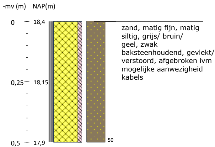
Boring 15 RD-coördinaten: 229894/475583
