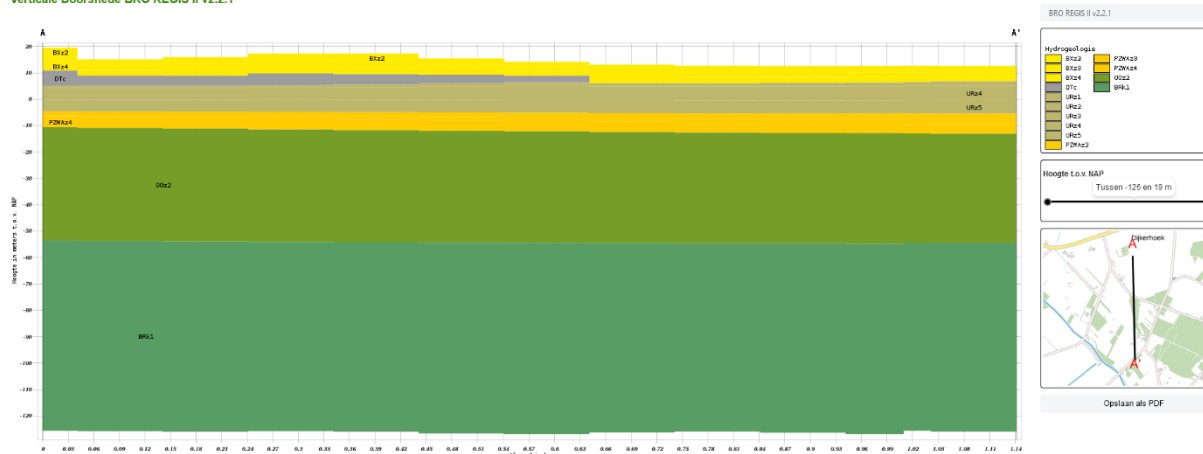
figuur 2: bodemopbouw
