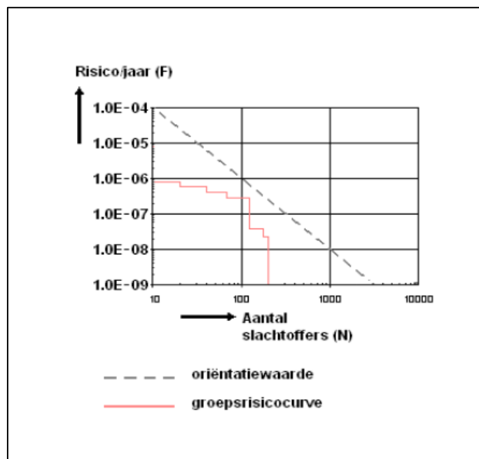
Figuur 4: groepsrisicografiek met orientatiewaarde
