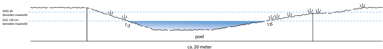
principeprofiel paddenpoel (zuid-noord)
