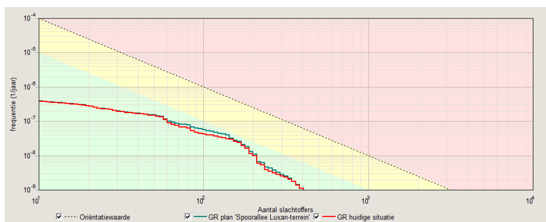
Figuur 4.1 Groepsrisico voor de realisatie van het plangebied 'Spoorallee – Luxan-terrein Elst'.
