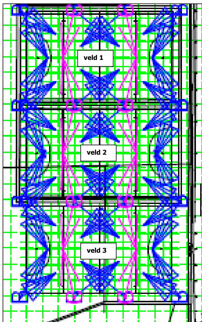
Figuur 2: ontwerp lichtmasten en uitstralingsrichting armaturen.
