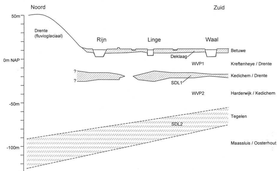
Afbeelding 4.1 Schematische bodemopbouw
