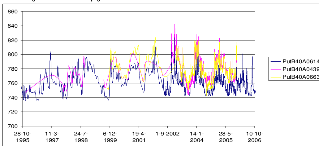
Afbeelding 4.5 Verloop grondwaterstanden
