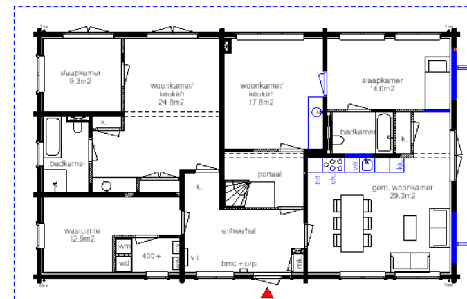
Begane grond, Finse woning NIEUW bvo: 168m 2
