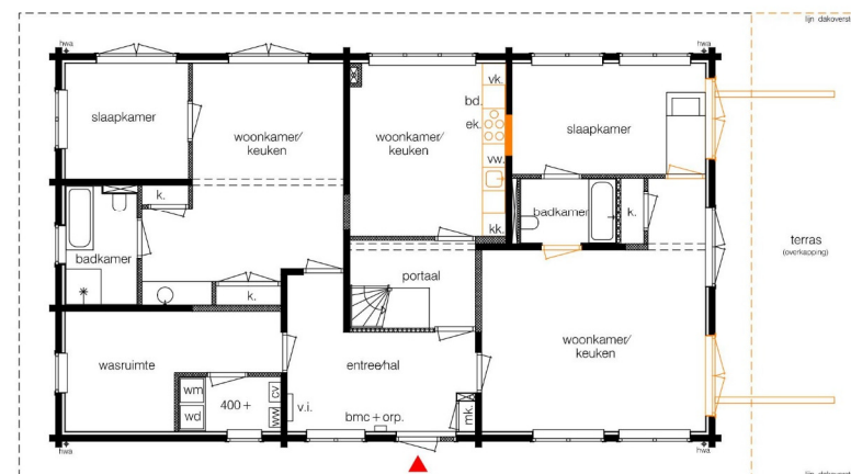
Begane grond, Finse woning BESTAAND bvo: 168m 2
