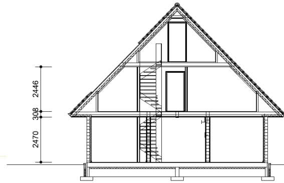
Doorsnede, Finse woning Bestaand
