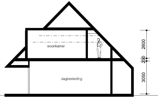
Doorsnede, Finse woning Nieuw
