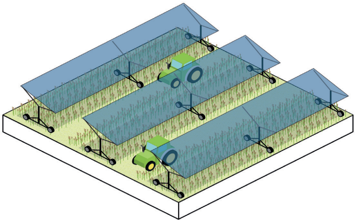
Transparante verrijdbare panelen maken landbouwproductie onder panelen mogelijk
