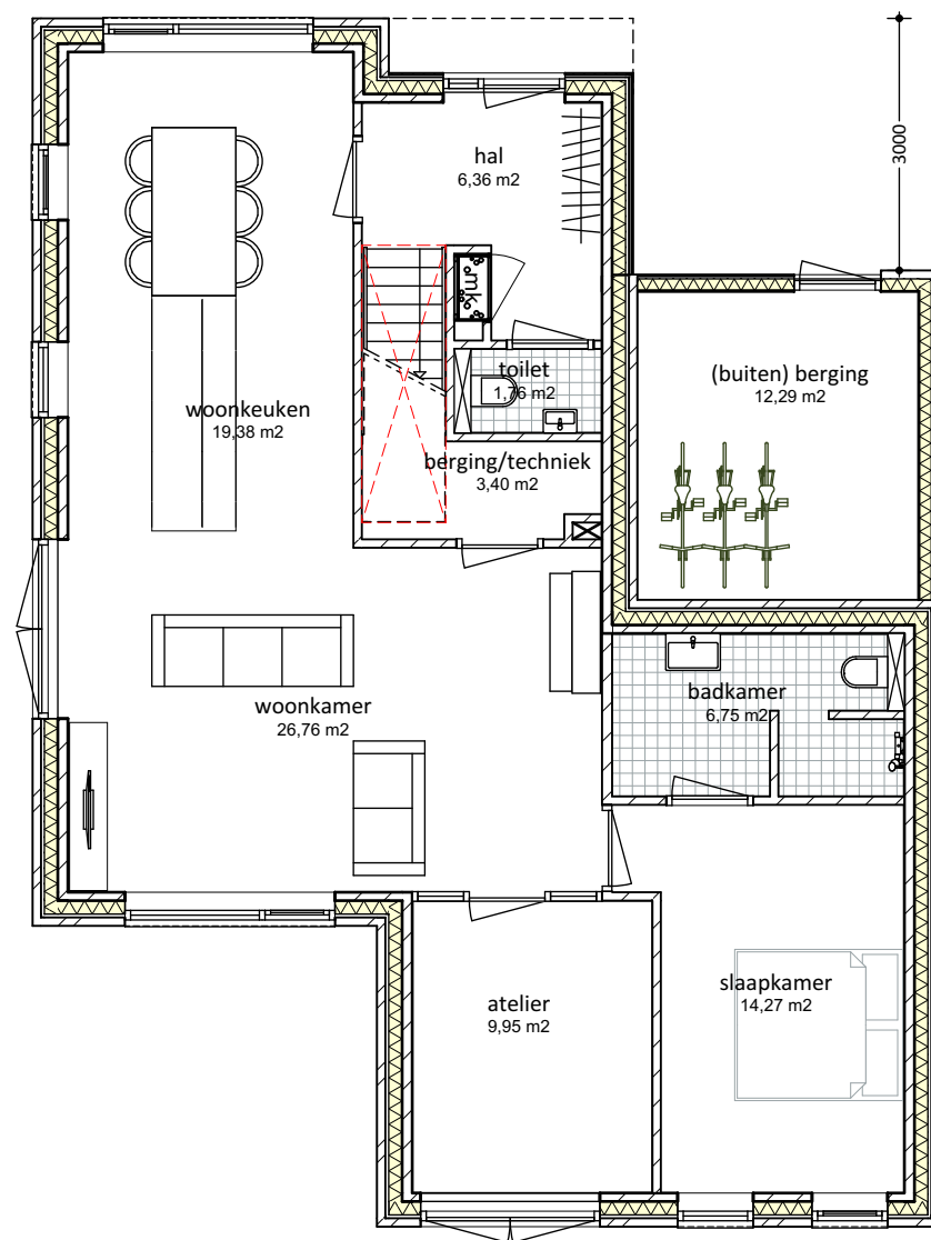
BEGANE GROND
