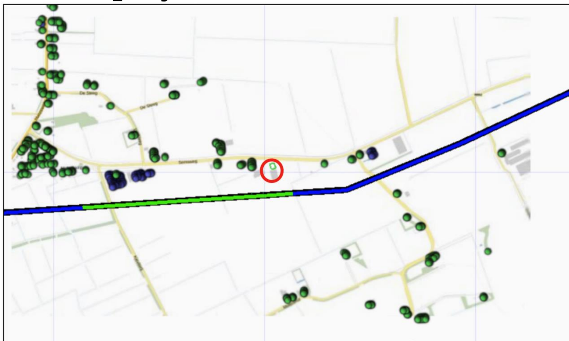
Figuur 4.2 Kilometer leiding behorende bij de maximale overschrijding van de FN-curve voor 7626_leiding-A-540-deel-1 van N.V. Nederlandse Gasunie
