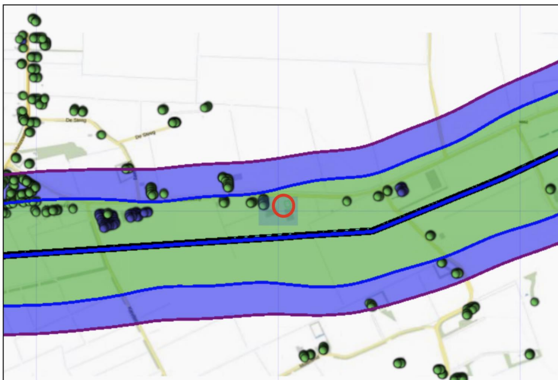
Figuur 3.1 Plaatsgebonden risico voor 7626_leiding-A-540-deel-1 van N.V. Nederlandse Gasunie
