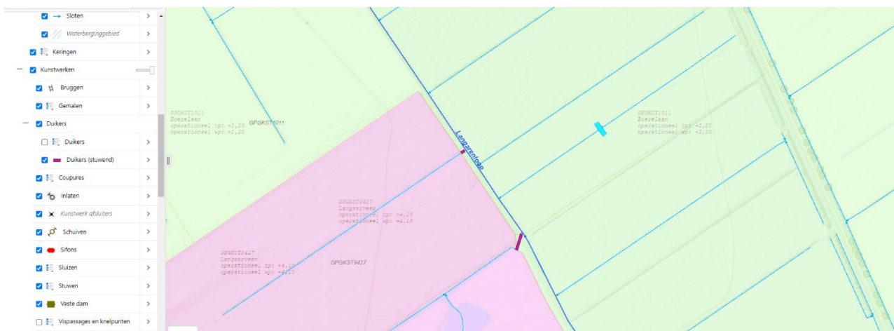
Figuur 7: Peilvakken behorende van het projectgebied (in het groen) en het peilgebied van Langaarsveen (Roze). De dikkere roze strepen geven de locaties van stuwende duikers aan. (Bron: Waterschap Noordzijlvest, 2021).
