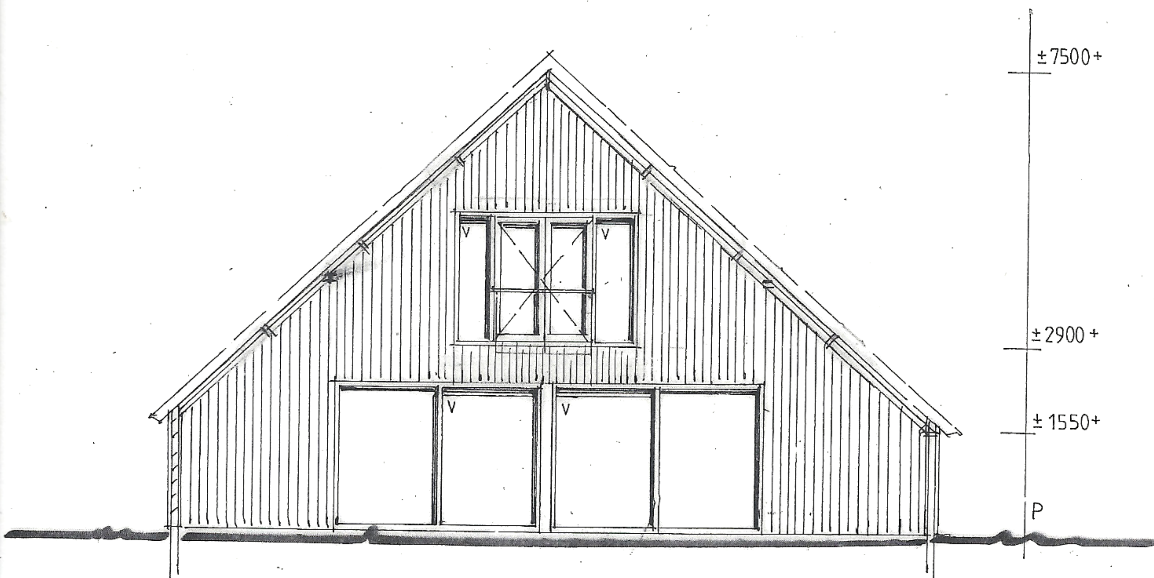
DOORSNEDE D_D
