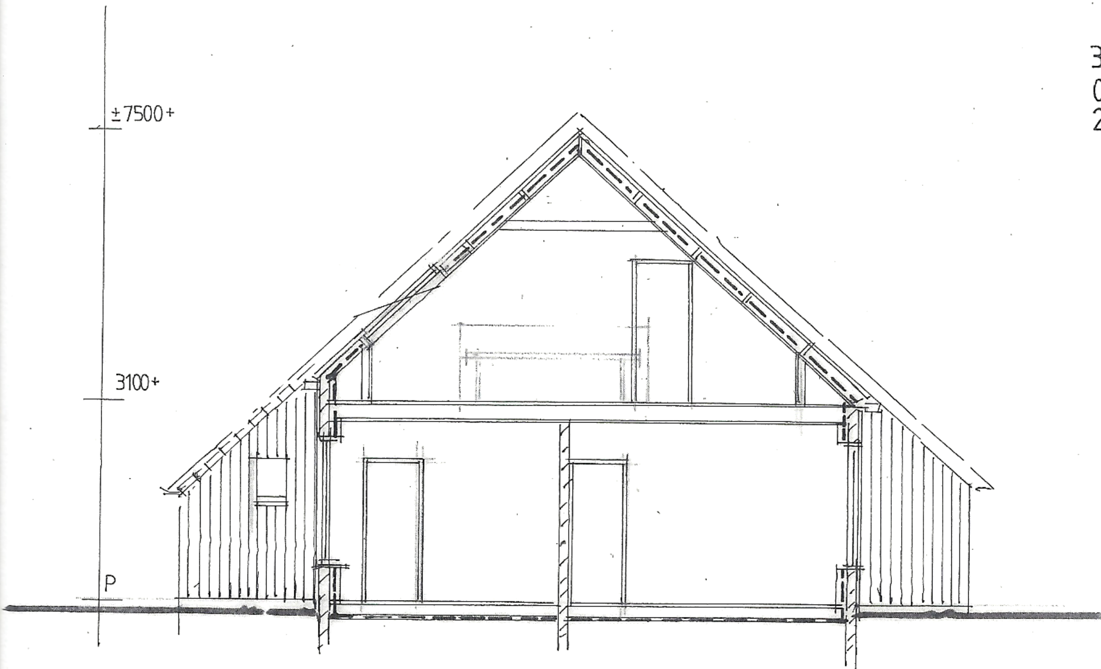
DOORSNEDE C_C
