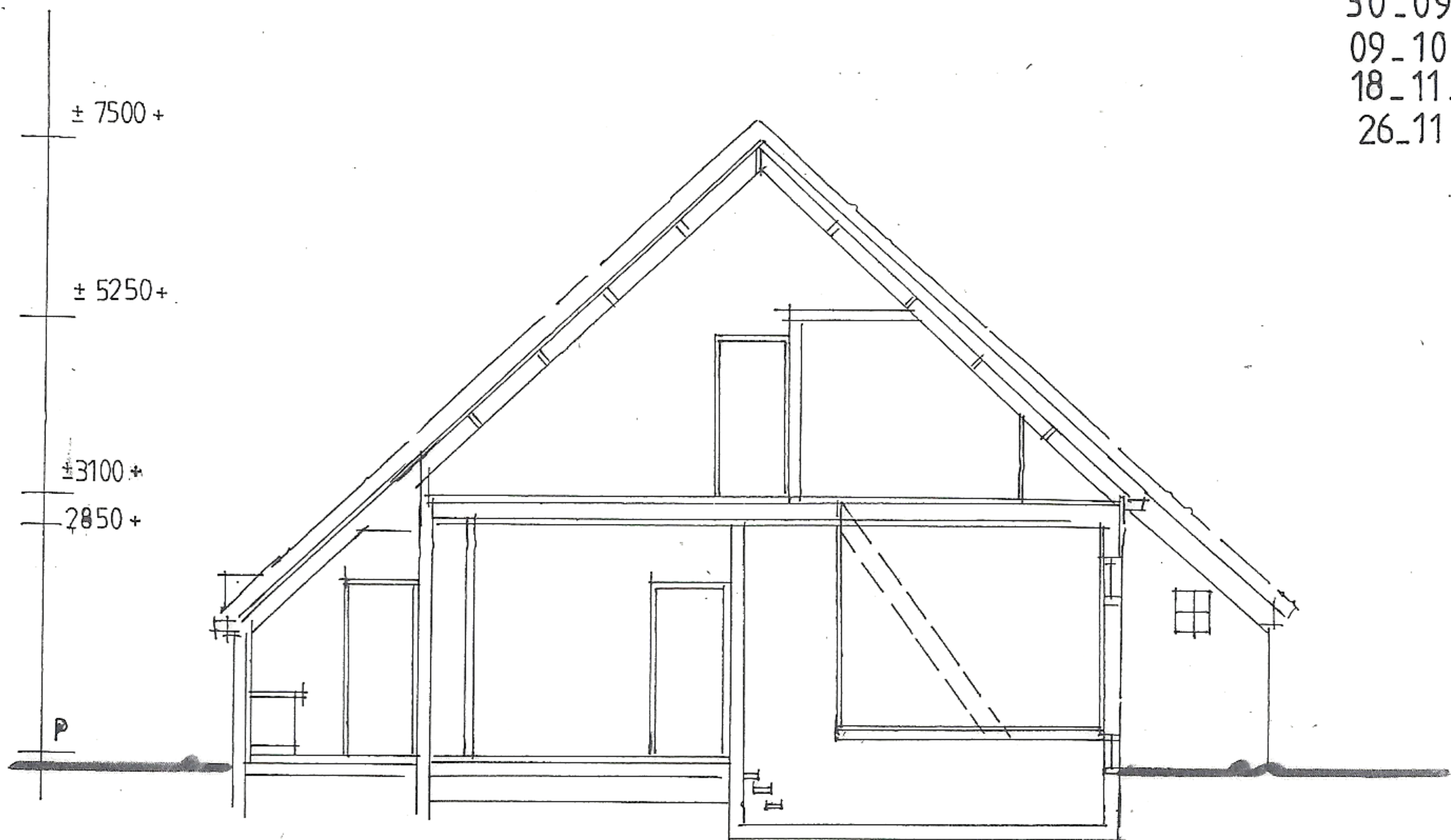
DOORSNEDE A-A
