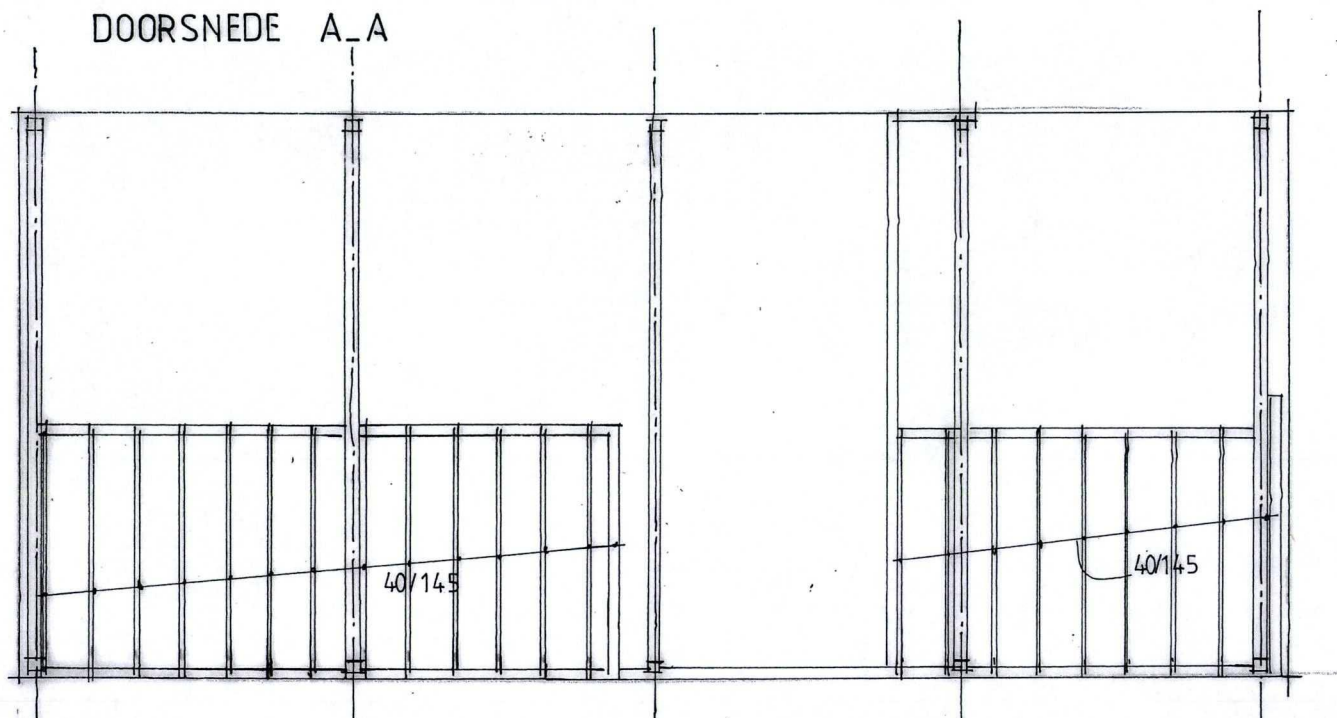
ZOLDER VLOER
