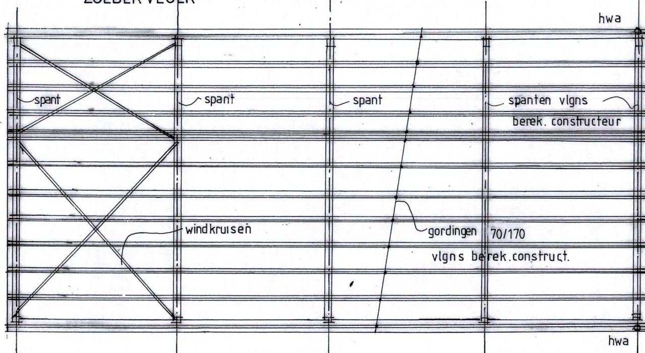
KAPPLAN
