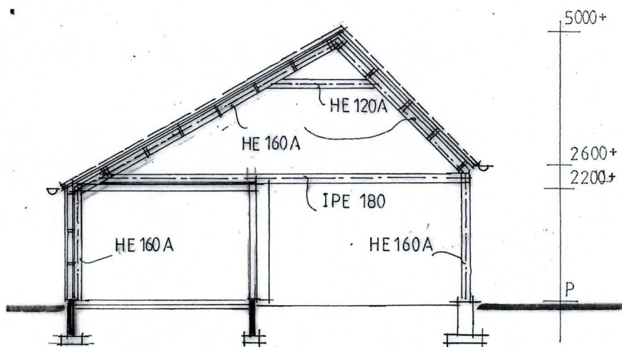
DOORSNEDE A-A
