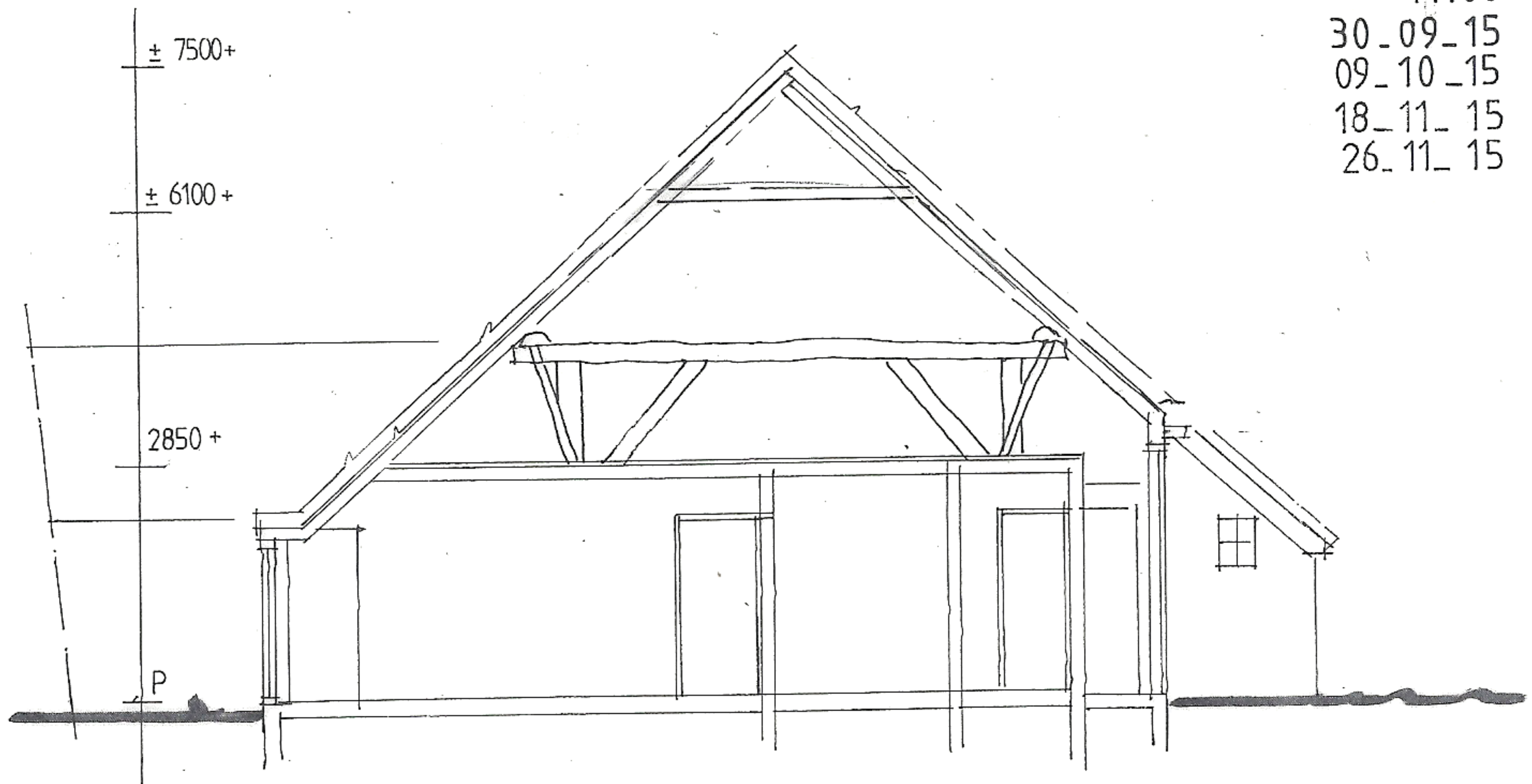
DOORSNEDE D-D
