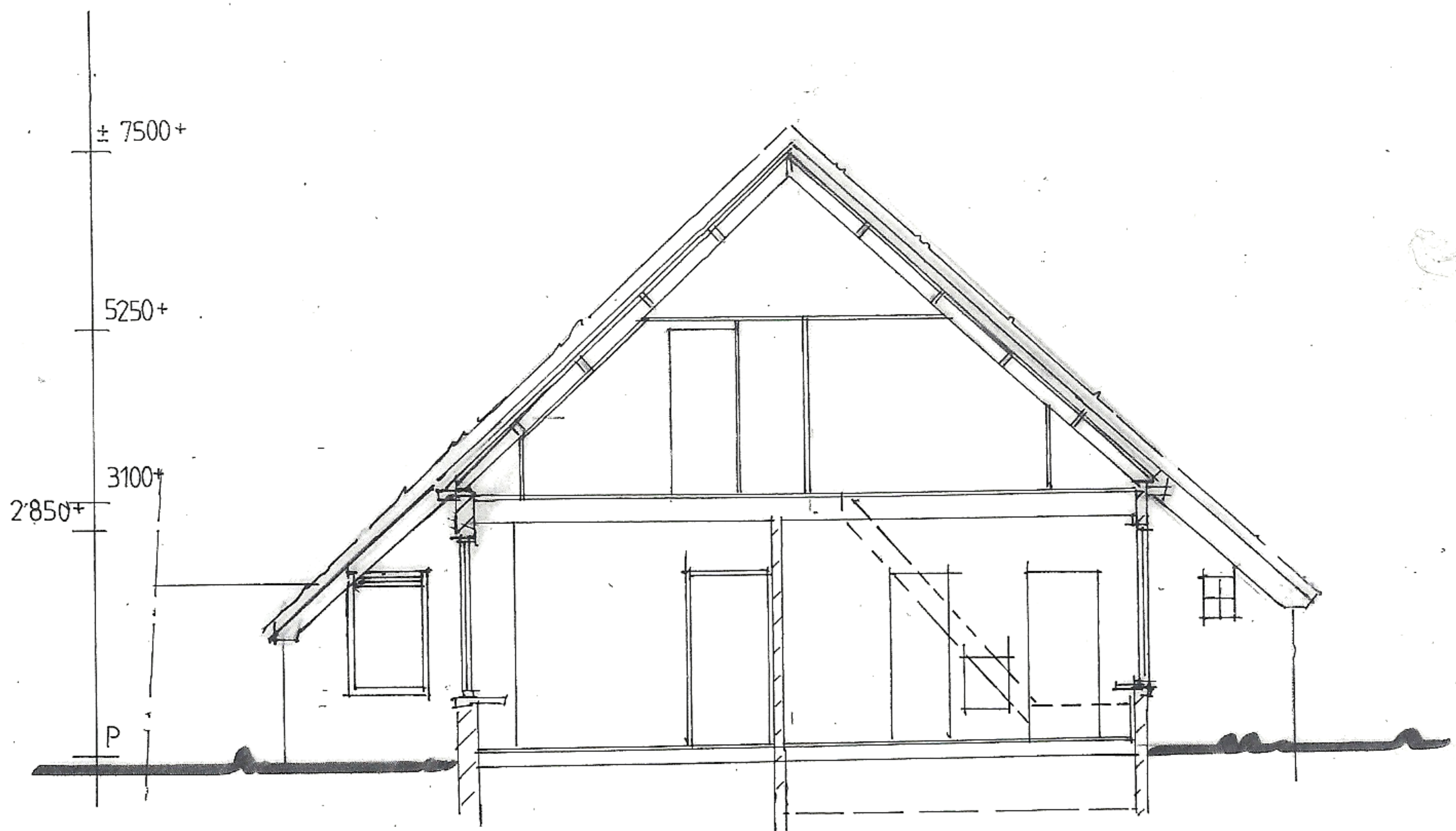
DOORSNEDE A-A
