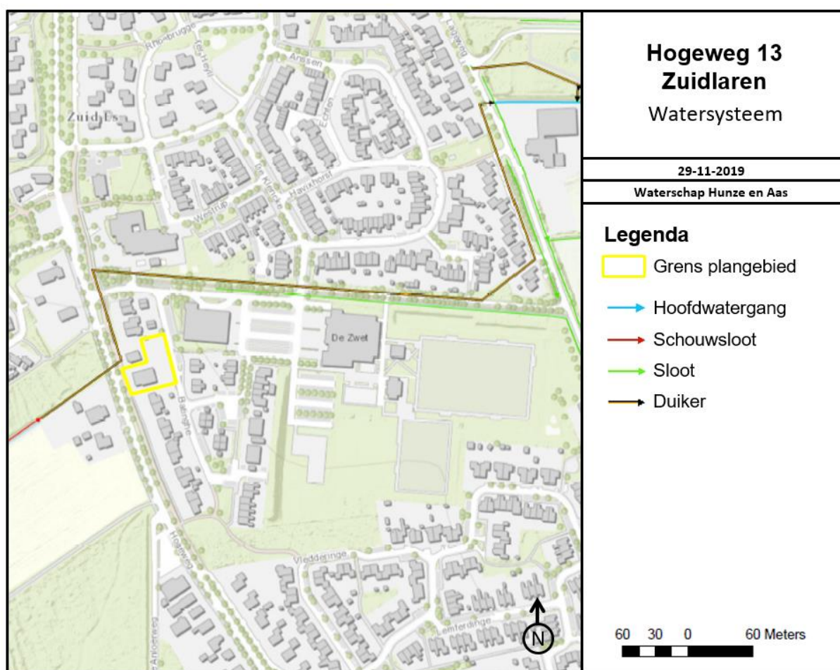
Figuur 1: oppervlaktewatersysteem
