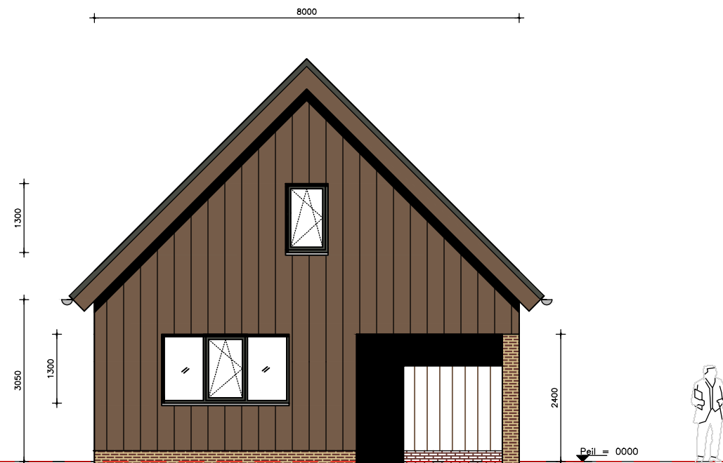
Rechterzijgevel
