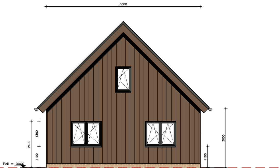
Linkerzijgevel
