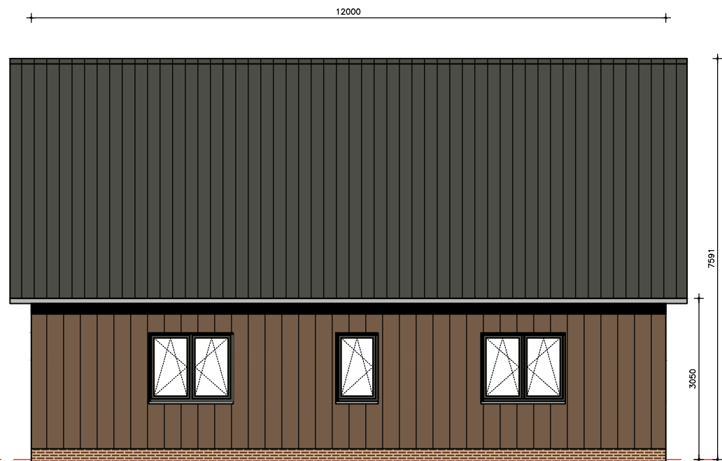
Straatgevel
