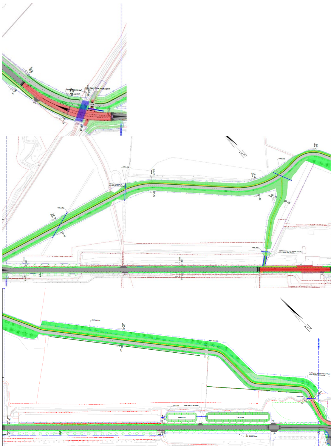
Figuur 1: Ontwerp van het vrijliggend fietspad.
