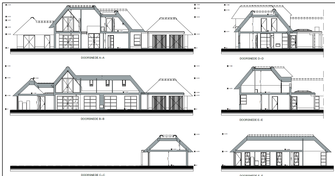
Afbeelding 5: Doorsneden
