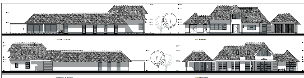
Afbeelding 4: Gevels
