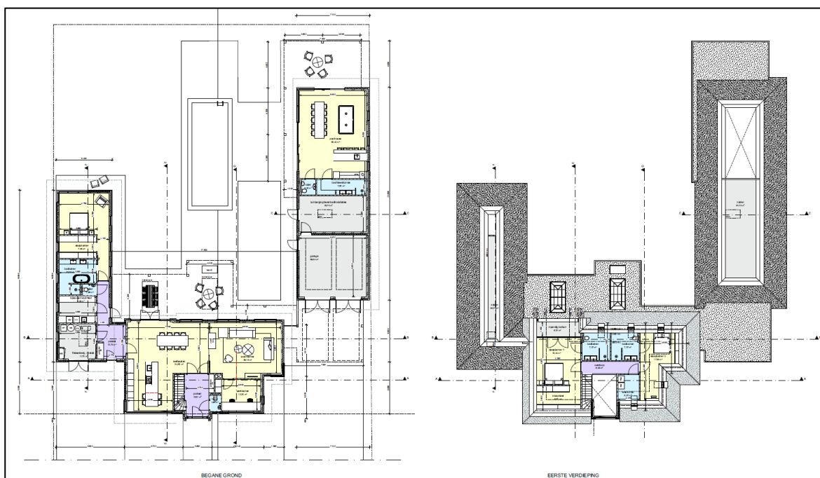
Afbeelding 3: plattegronden
