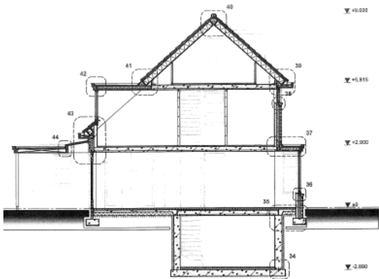
DOORSNEDE B-B
