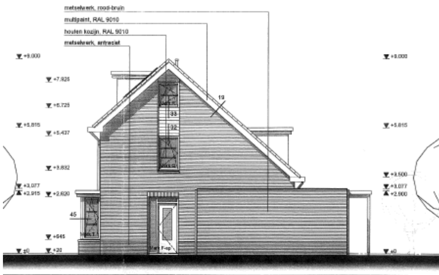
RECHTER ZIJGEVEL
