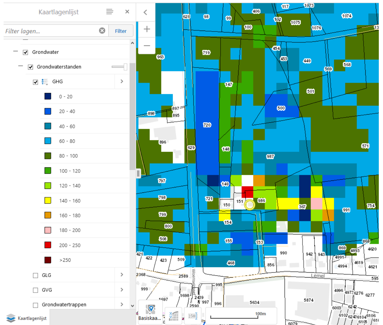
Figuur 1 | Gemiddelde hoogste grondwaterstand (GHG)
