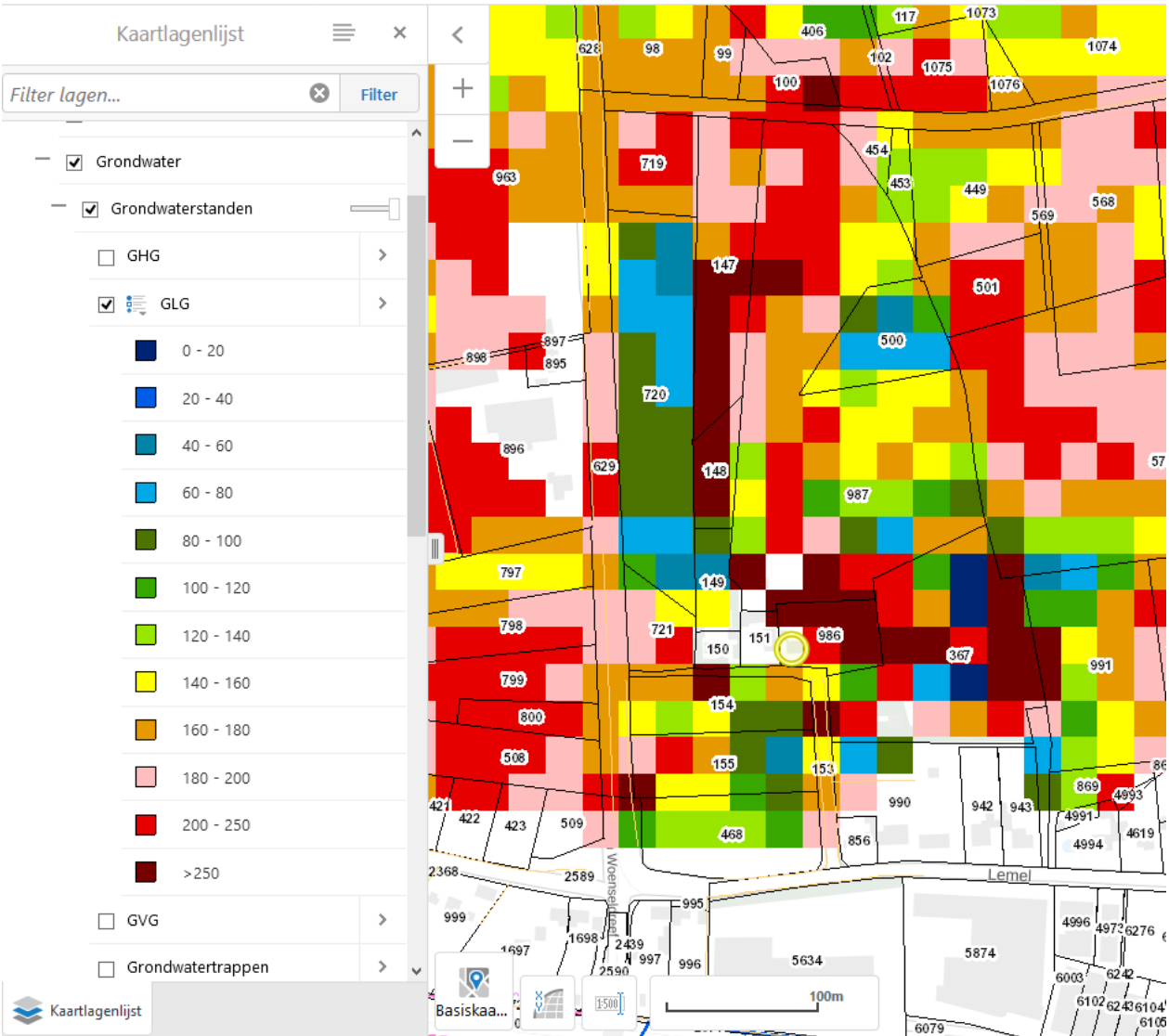
Figuur 2 | Gemiddelde laagste grondwaterstand (GLG)
