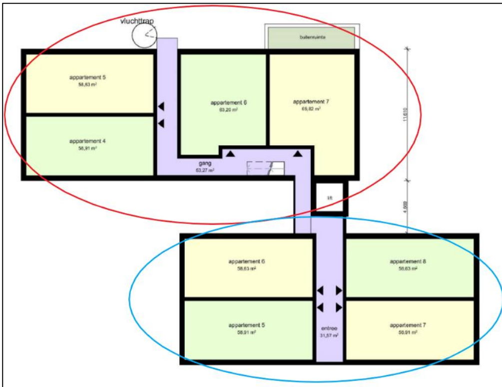
Afbeelding 4: schets Wenshuys eerste verdieping bestaand en nieuw
