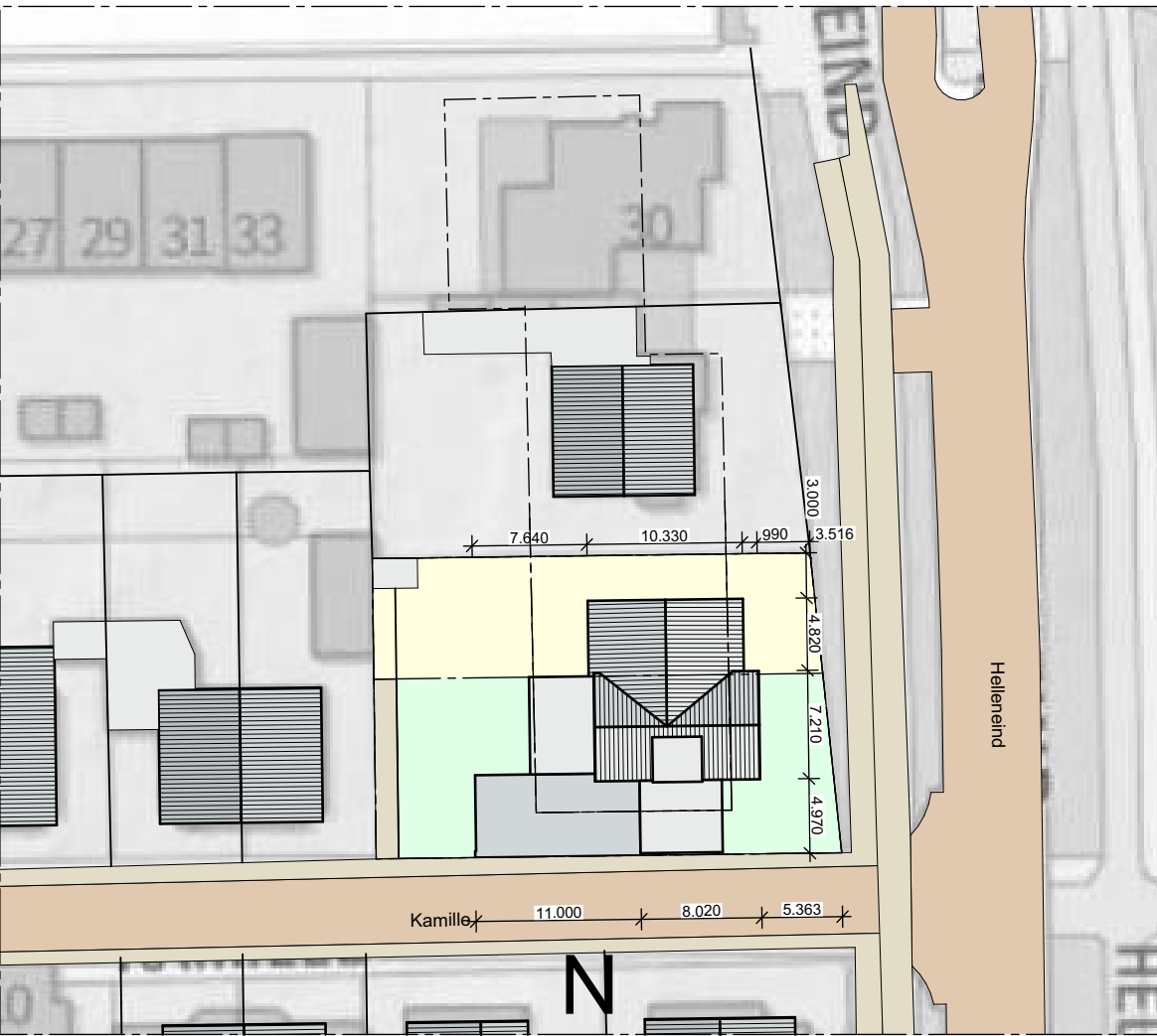
SITUATIE Gemeente : Bladel Sectie : G Nr. : 1274 Schaal : 1 : 50
