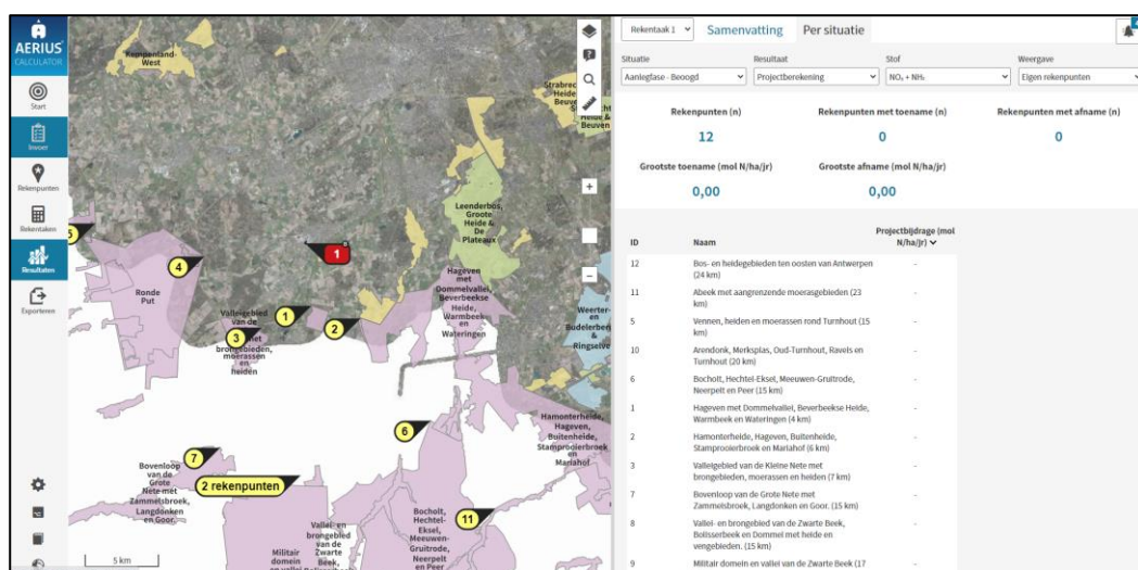
Afbeelding 1: Ligging en rekenresultaten eigen rekenpunten aanlegfase
