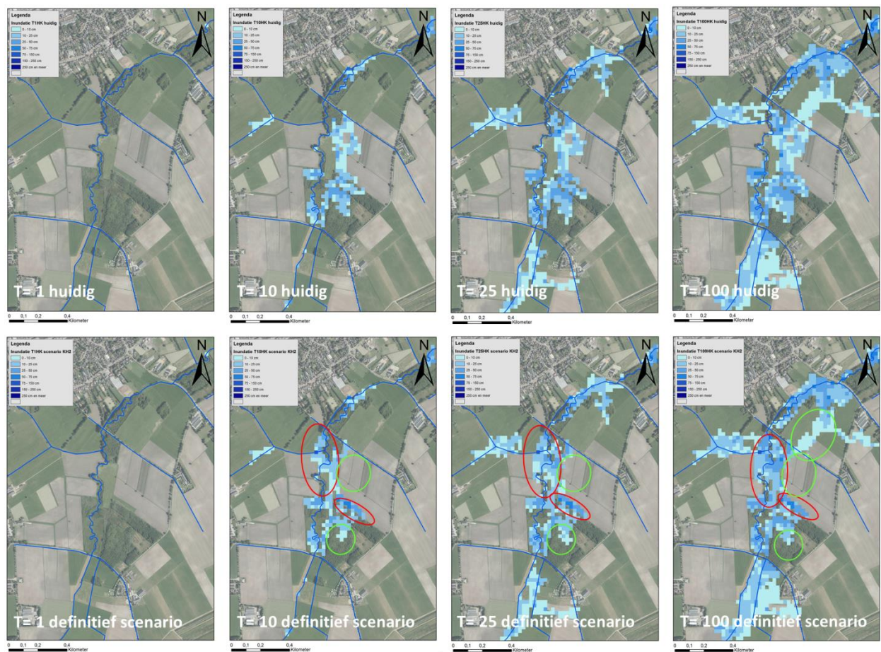
Figuur 1.5: Berekende inundaties in huidig klimaat (boven) en in definitief scenario (onder) voor herhalings tijden T=1, 10, 25 en 100. Met rode cirkels is toename inundatie aangegeven. Met groene cirkels afname inundatie
