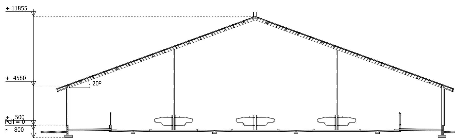
Doorsnede 4
