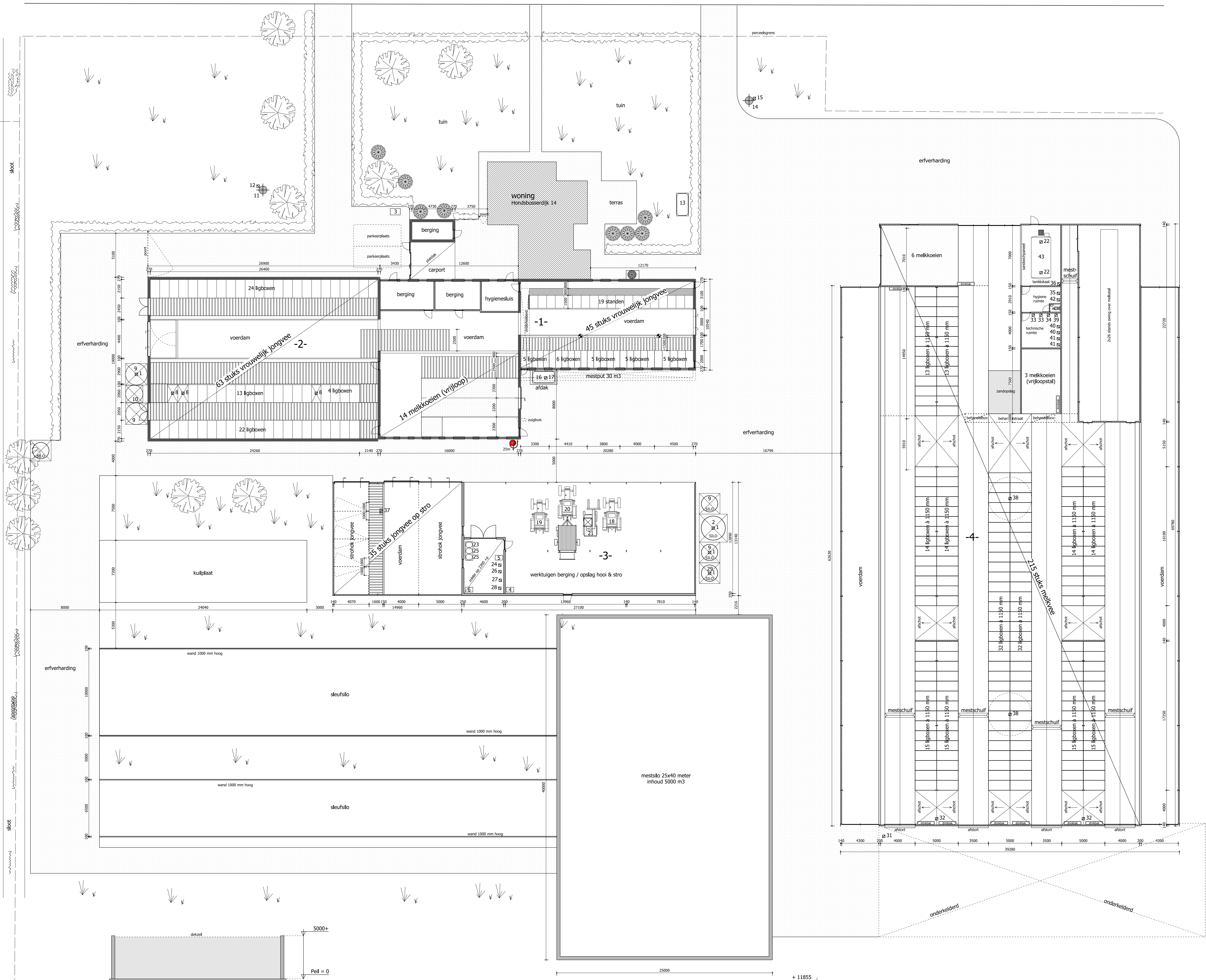
Doorsnede mestsiilo
