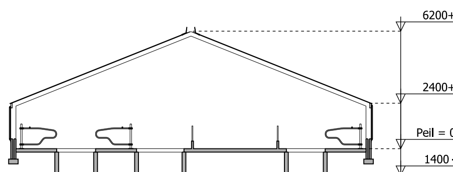
Doorsnede 2
