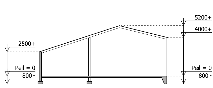
Doorsnede 3
