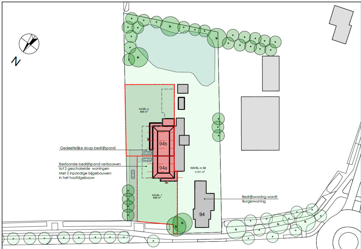
Afbeelding 2: Plattegrond beoogd
