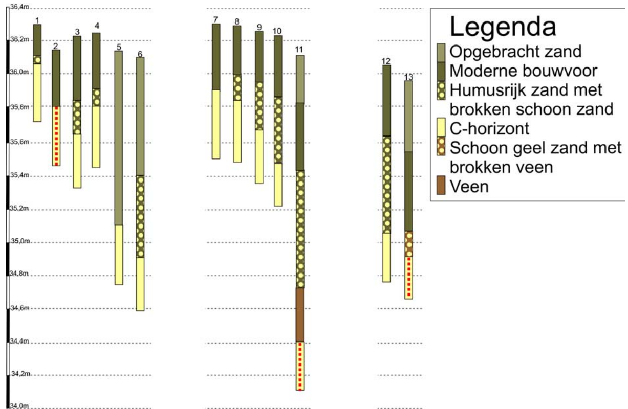
Figuur 14: Boorprofielen
