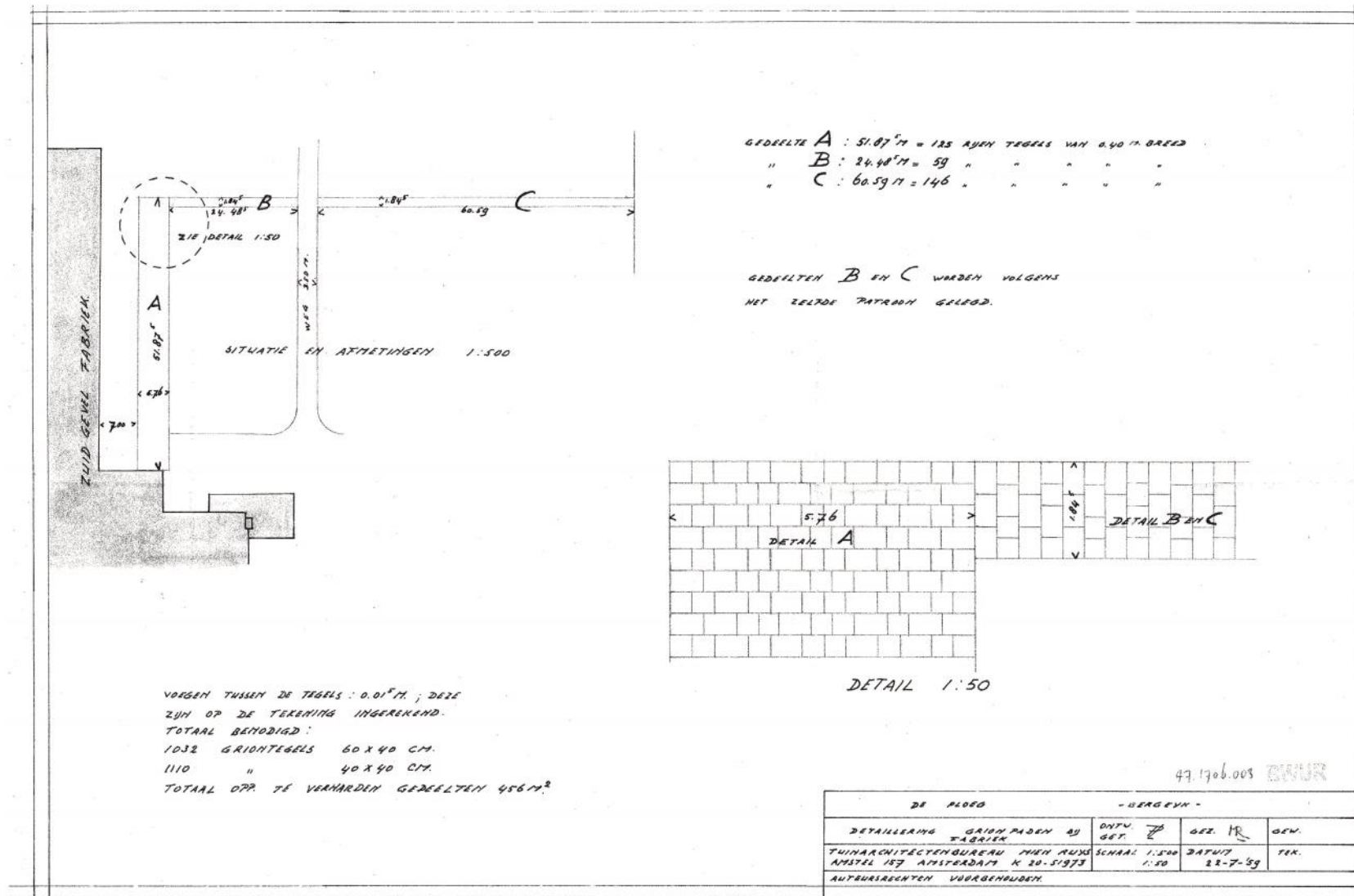
Detailering patroon Griontegels bij De Ploeg; Buro Mien Ruys
