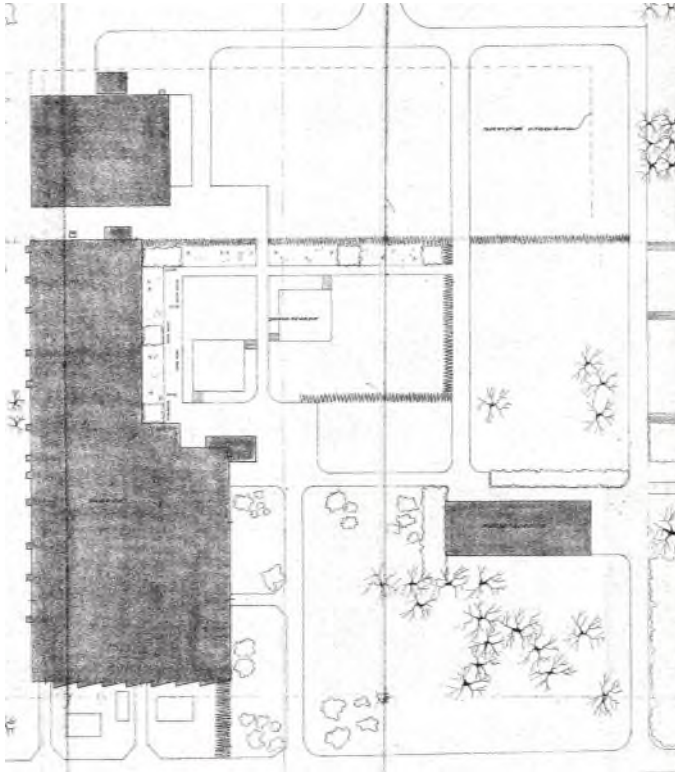
Uitsnede ontwerp Ploegpark, 04-05-1959, gewijzigd 29-08-1961; Buro Mien Ruys
