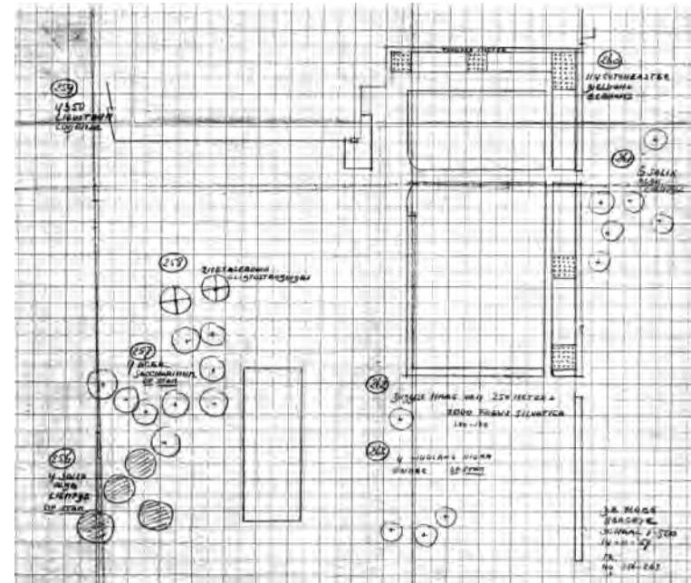
Beplantingsplan, 14-11-1959; Buro Mien Ruys
