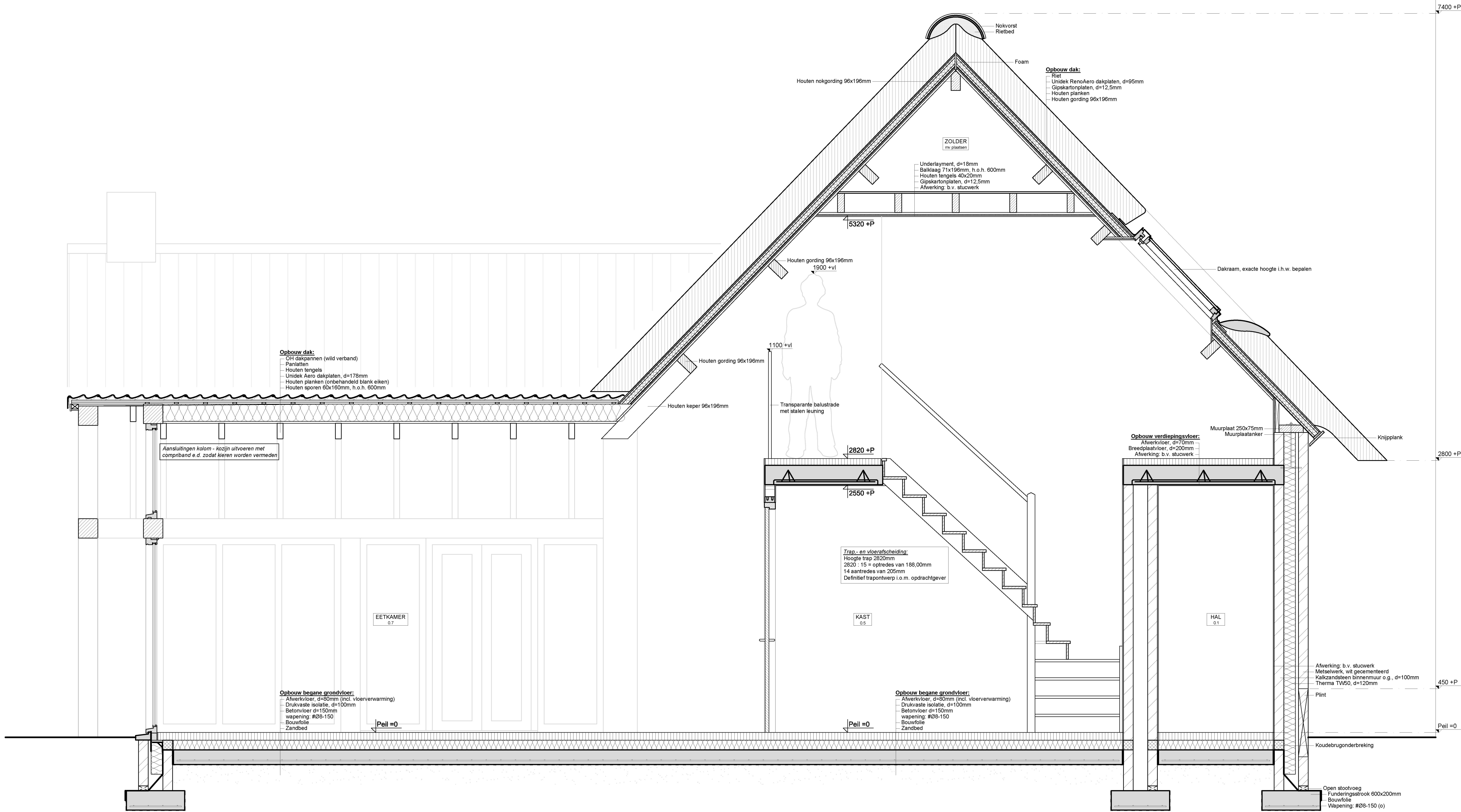
Doorsnede B-B
