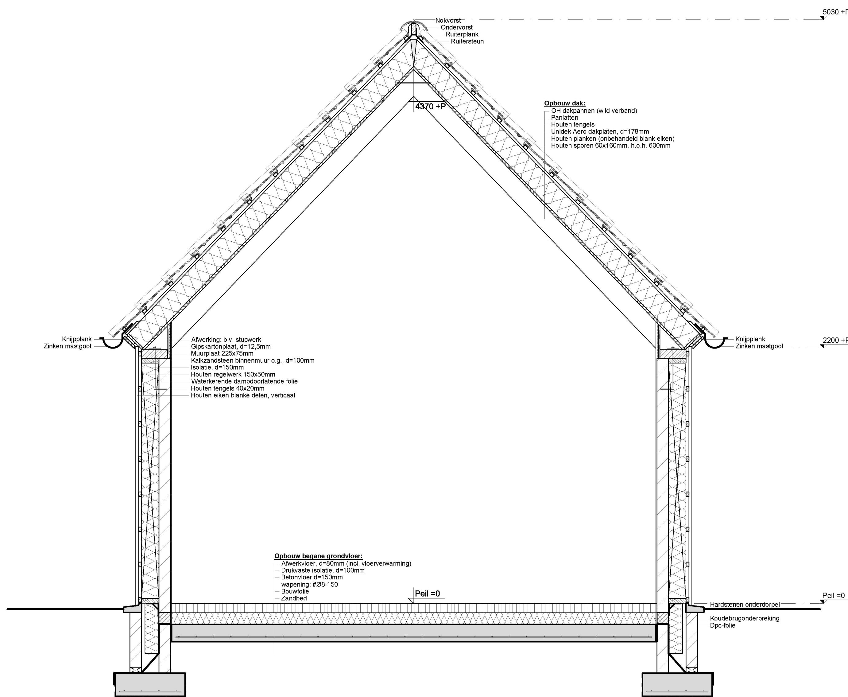
Doorsnede D-D
