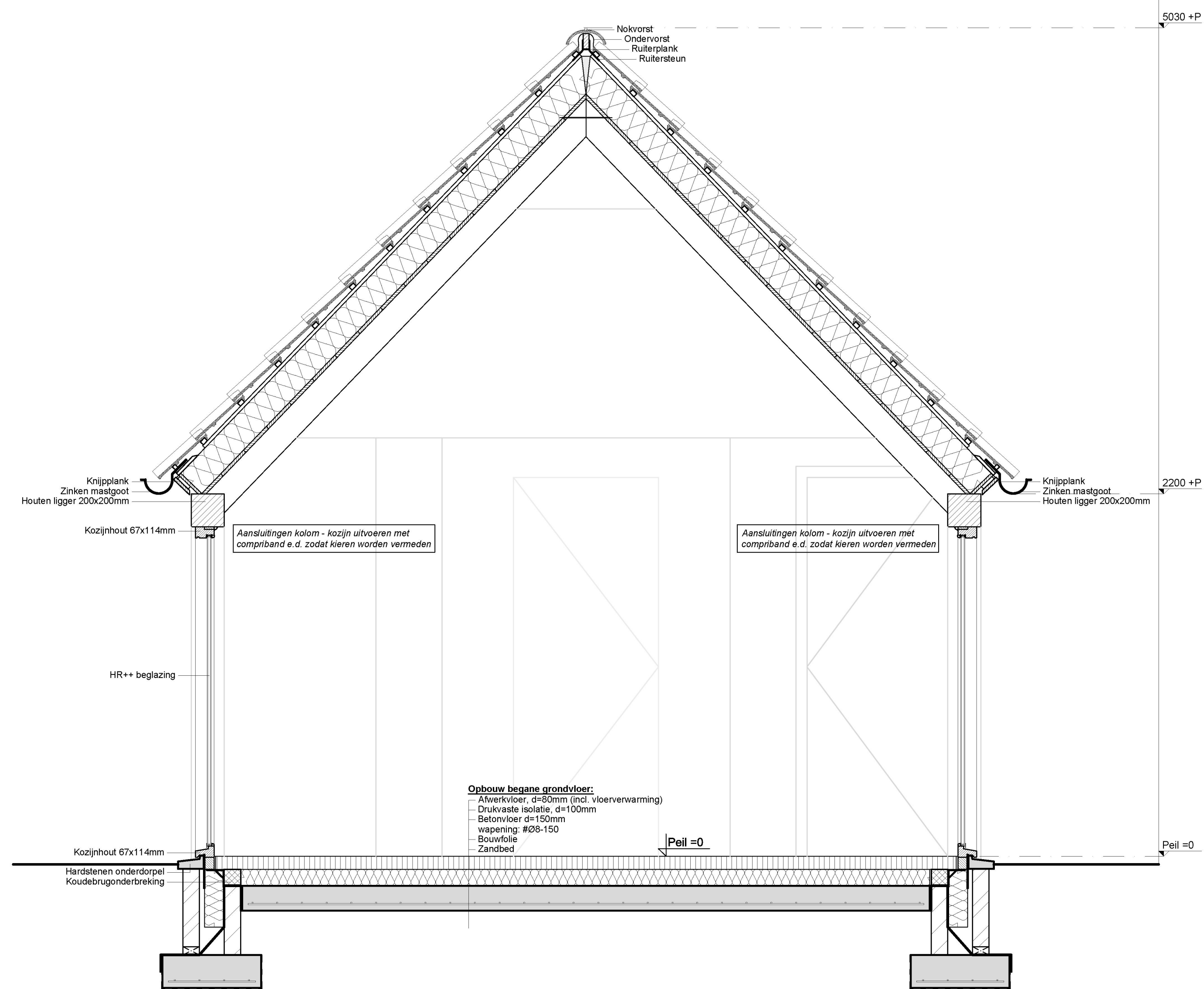
Doorsnede E-E
