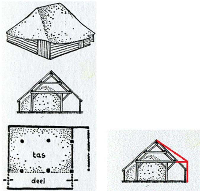
Schematische weergave van een Vlaamse schuur, met rechts in rood een schematische weergave van de tweede bouwphase.
