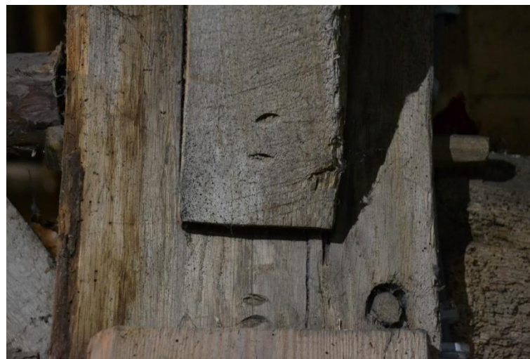
2 Gegutste ovaaltjes op de gebintstijl en het korbeel.
