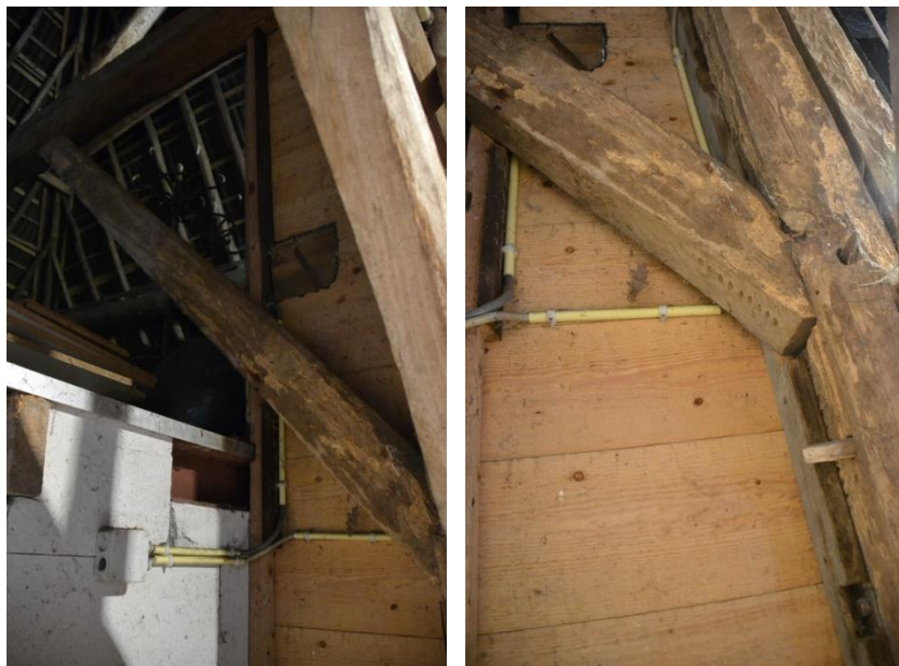
Links: korbeel dat gebintstijl 1a met gebintbalk verbindt. Rechts: detail korbeel.
