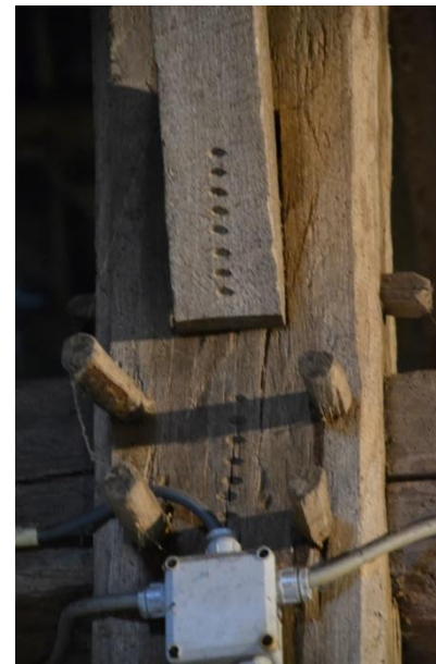
8 Gegutste ovaaltjes op de gebintstijl en het korbeel t.h.v. de middenbeuk.
