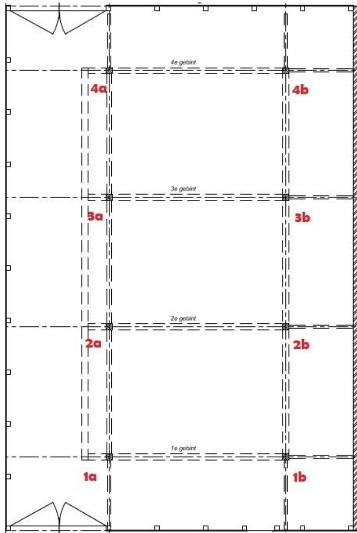
Voorbeeldplattegrond van een Vlaamse schuur met aanduiding van de gebintstijlen.
