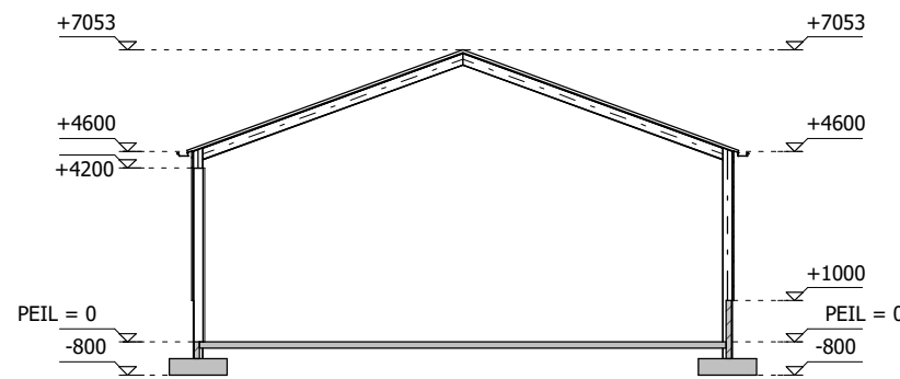
DOORSNEDE GEBOUW 2
