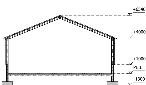
DOORSNEDE GEBOUW 3
