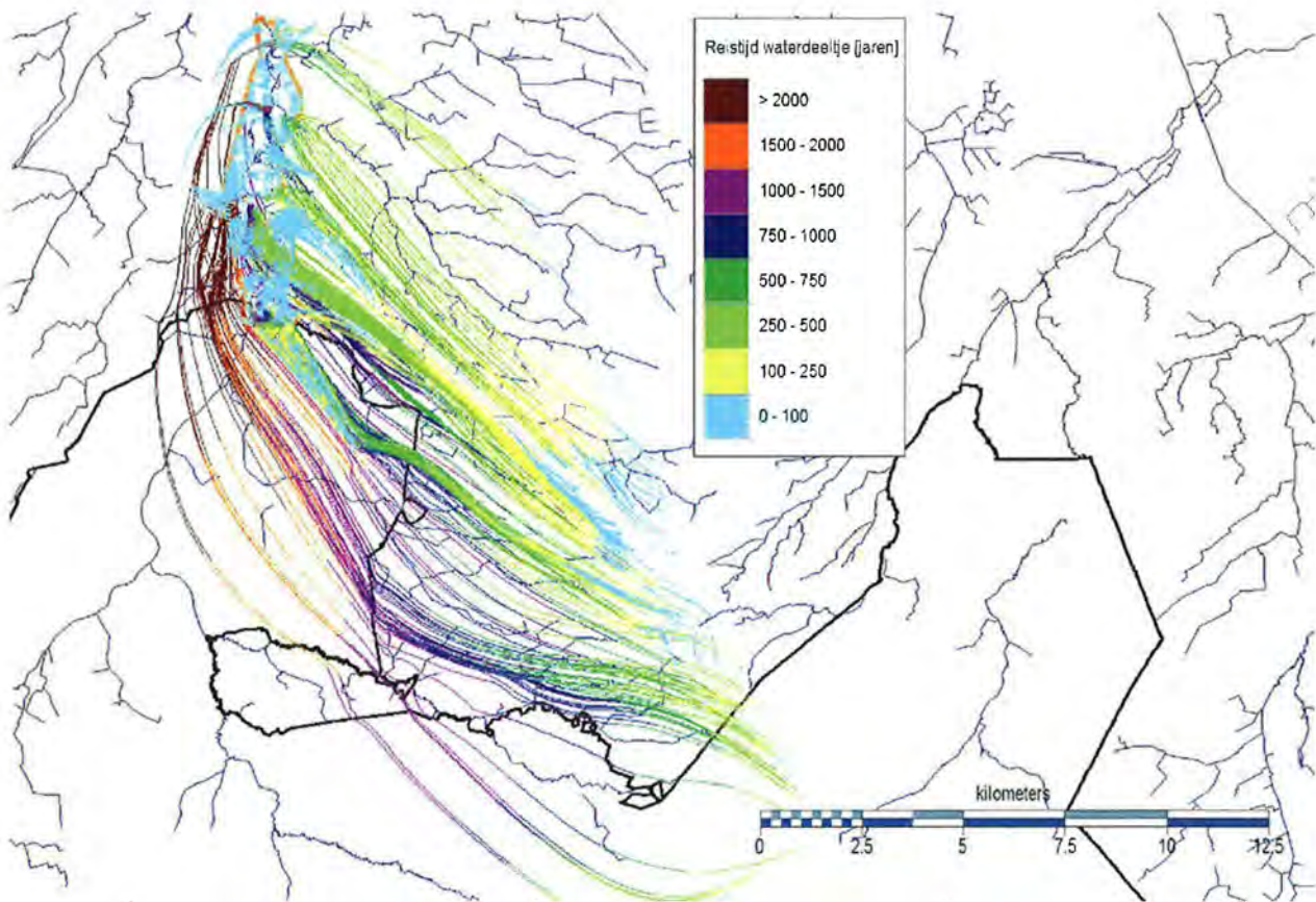
Figuur 23: Grondwaterstroming weergegeven met stroombanen door verschillende modellen naar het oppervlak in het Markdal.
