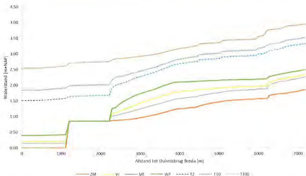
Figuur 40: Waterpeil voor verschillende maatgevende situaties van de Duivelsbrug (0 meter) tot de Oude Trambrug (10 km).
