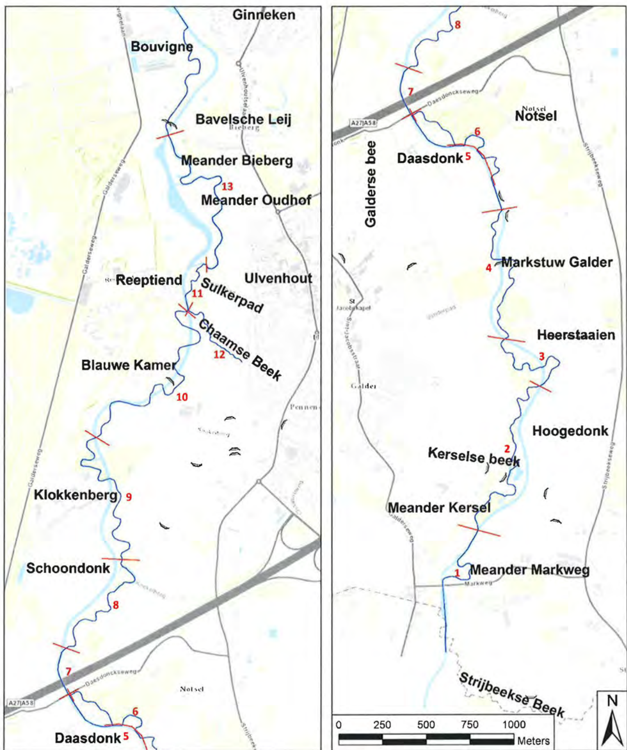
Figuur 46: Locaties van de trajecten waarvoor de stroomsnelheid is bepaald in het VKA
