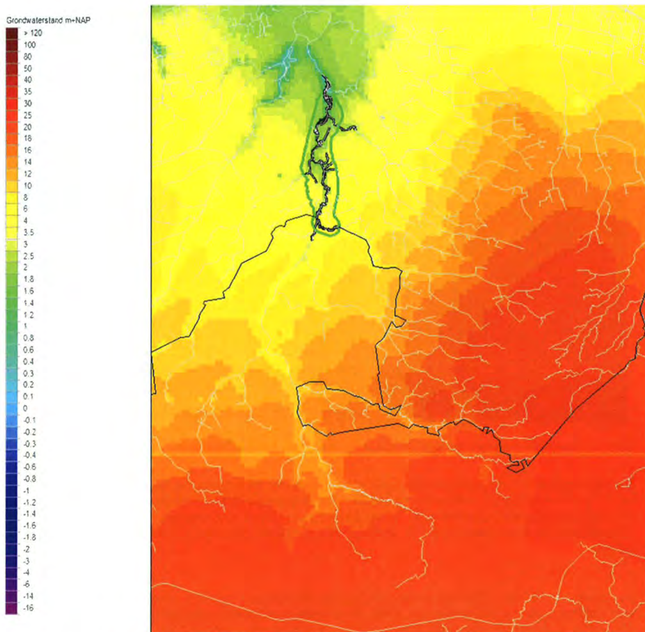
Figuur 6: Regionaal beeld van de grondwaterstand in m+NAP.
