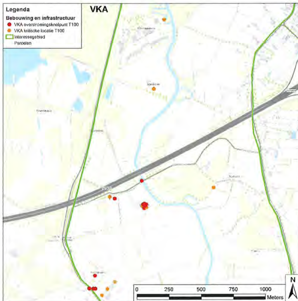
Figuur 45: Knelpunten wateroverlast VKA
