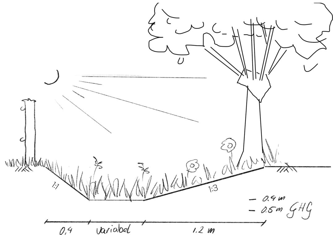
Principeprofiel infiltratiegreppel
