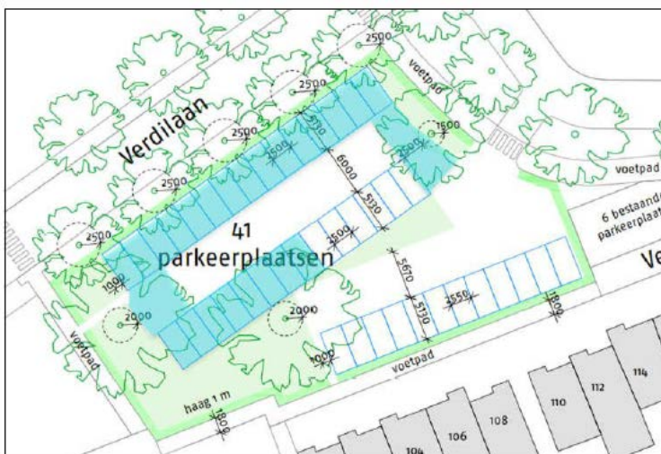
Afbeelding 21: Aangepast ontwerp (blauw: Permavoid fundering)
